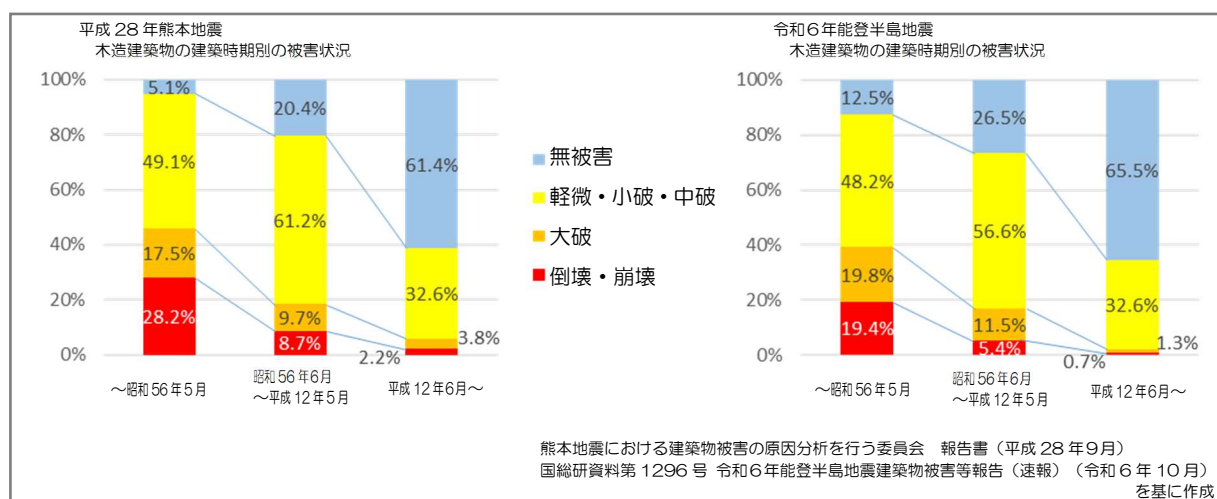
図 2-2 木造建築物の建築時期別の被害状況
