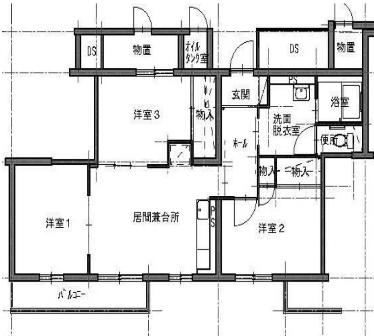
(間取りは、3LDKの一例です。)
