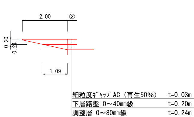
摺付部断面図 1 : 100
