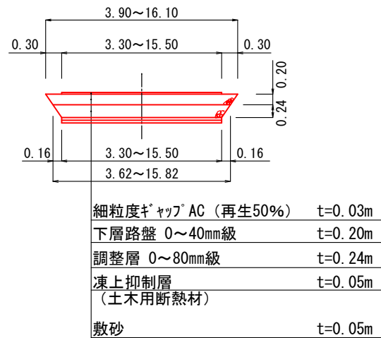
土工定規図 ② 1 : 100
