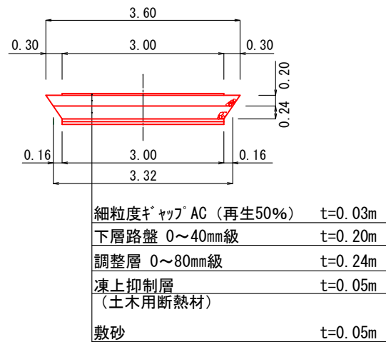
土工定規図 ① 1 : 100
