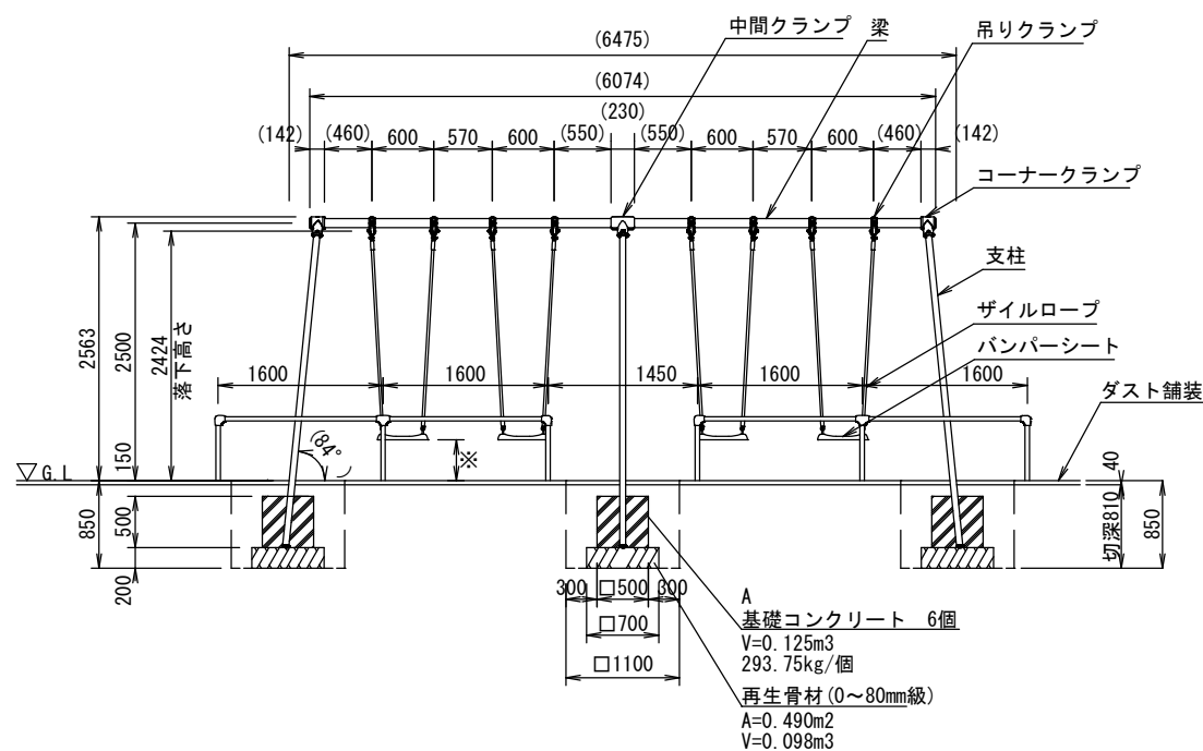
立面图 S=1/40
