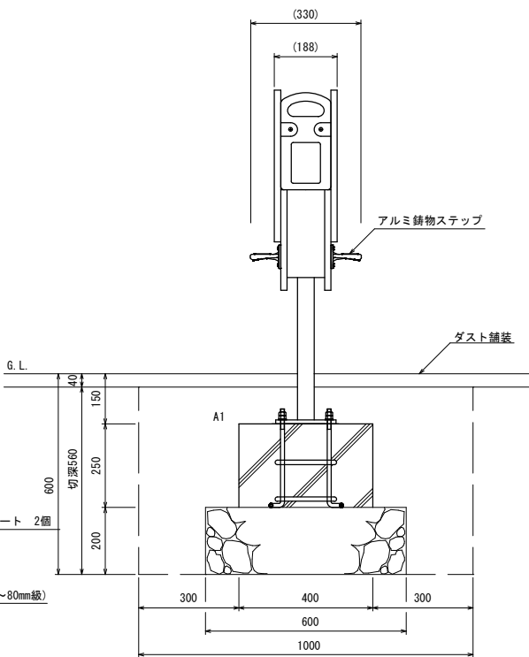
立面図
