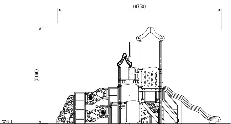
B立面図 S=1/50
