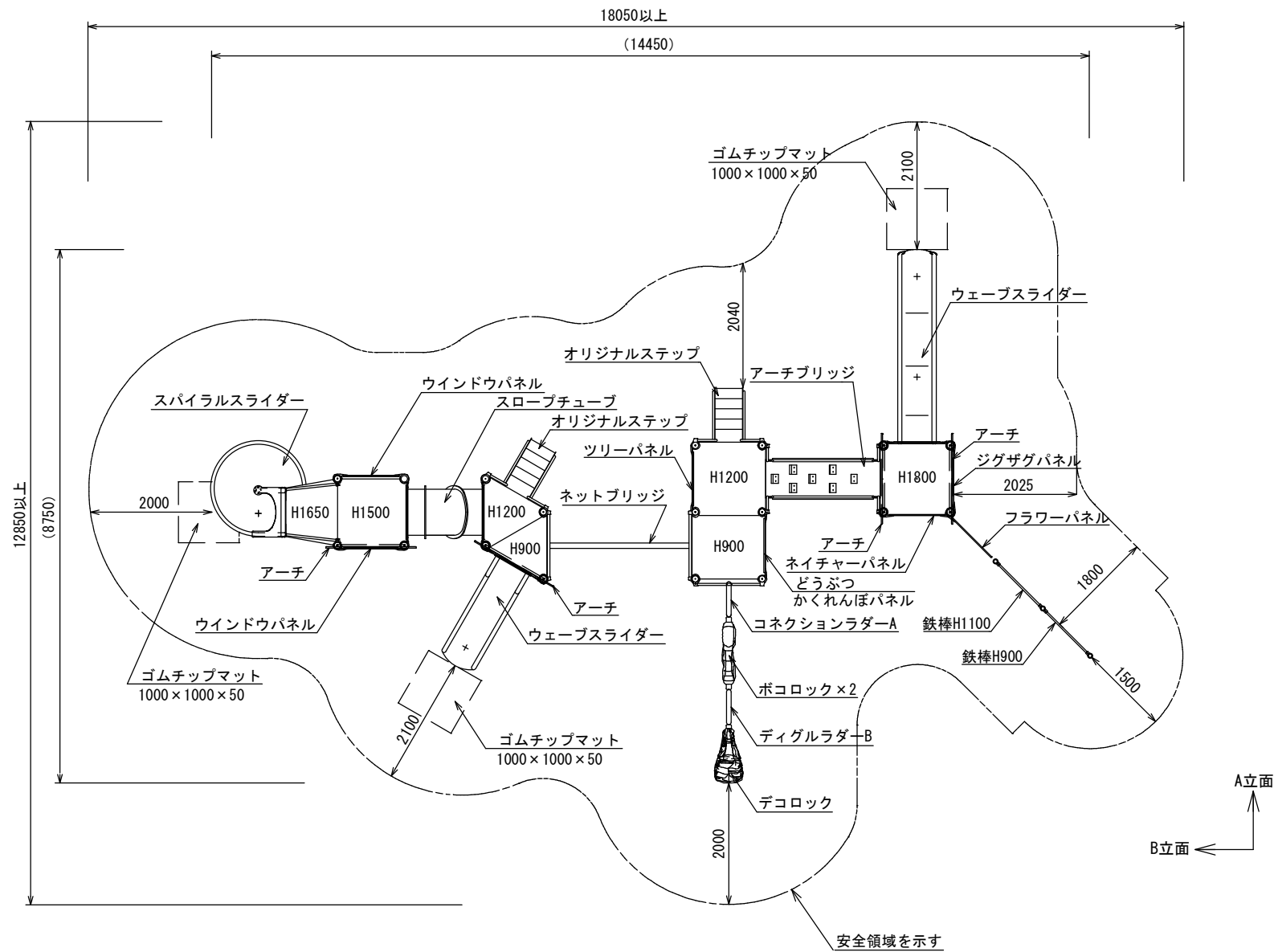
平面図 S=1/50
