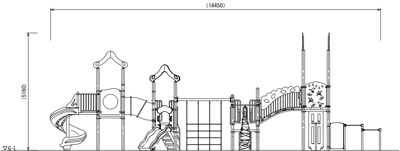
A立面図 S=1/50
