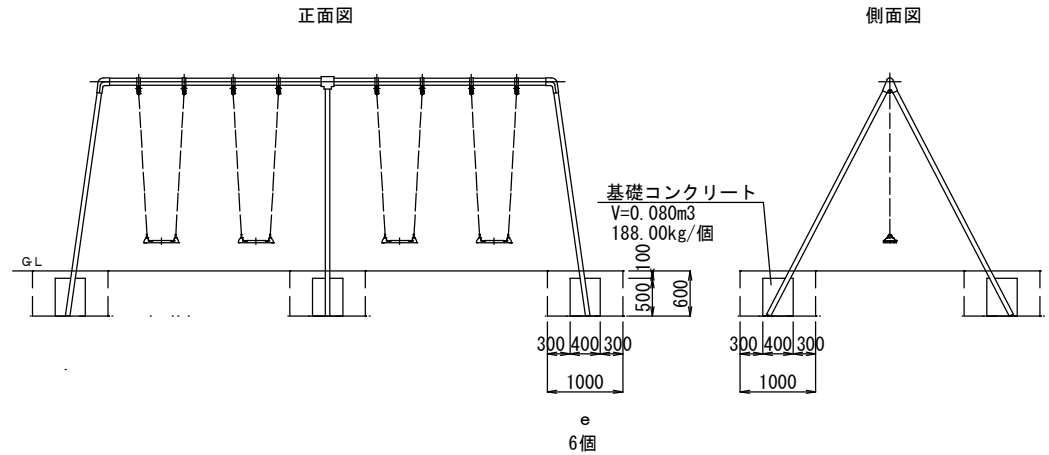
4連ブランコ基礎 1/50
