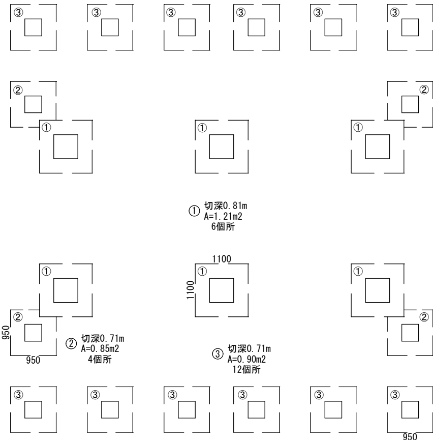
基礎状図 S=1/40
