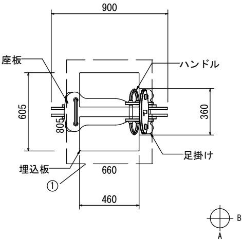
平面図 1/15
