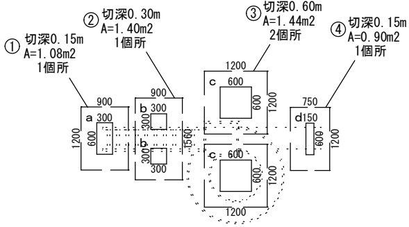
1回転式滑り台基礎 1/50
