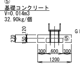
滑り台正面
