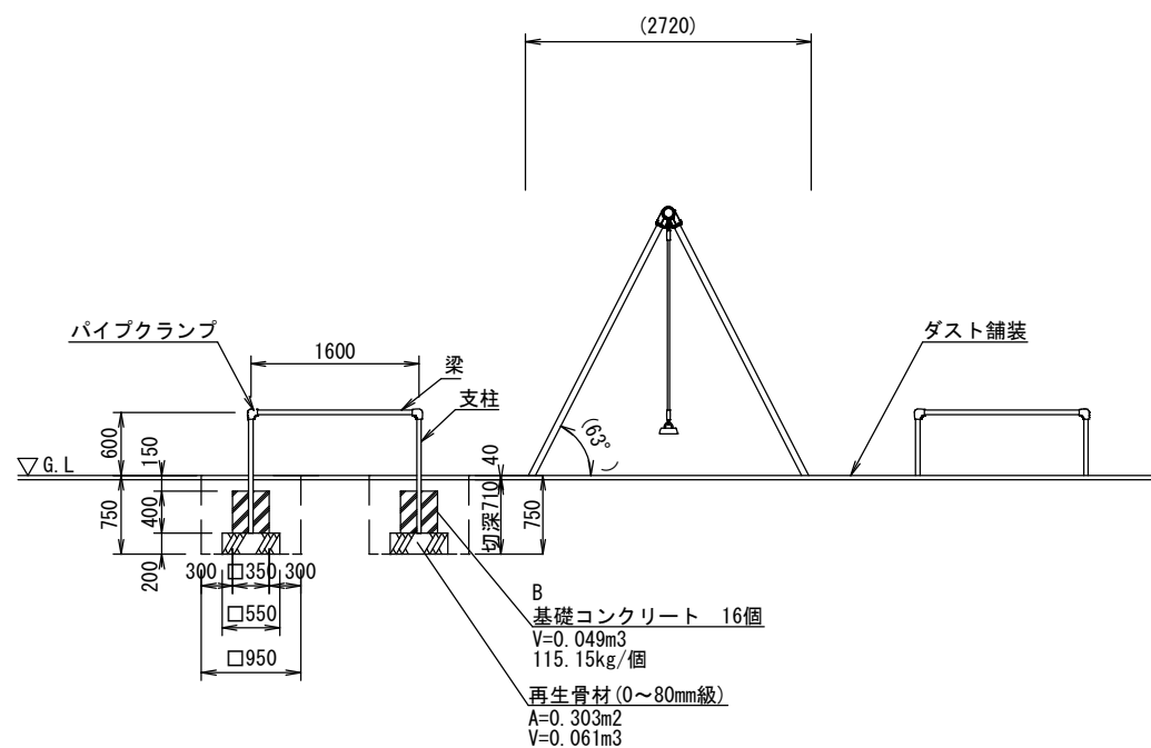
側面図 S=1/40
