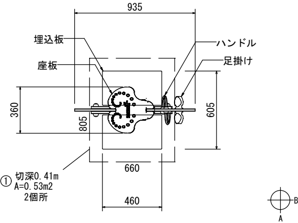
平面図 1/15
