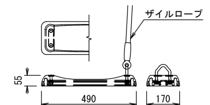
バンパーシート詳細図 S=1/10
