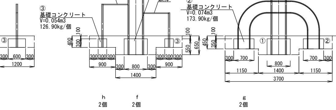
鉄棒側面
