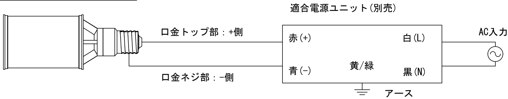
LEDランプ結線図
