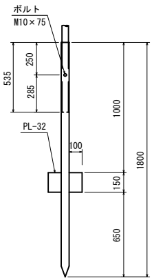
基礎管 S=1:20
