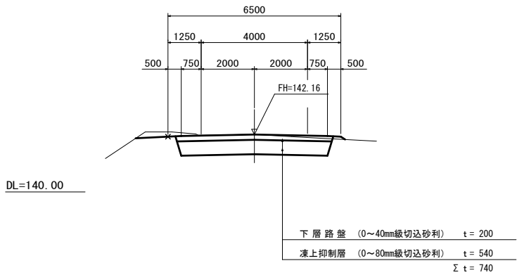
B-B断面図 S=1:100
