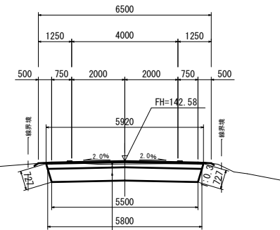
D-D断面図 S=1:100
