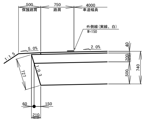
路肩詳細図 S=1:25
