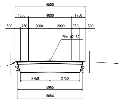
C-C断面図 S=1:100
