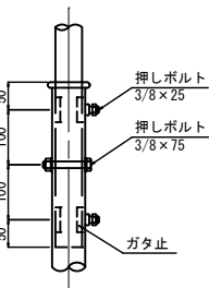
ジョイント部 S=1:5
