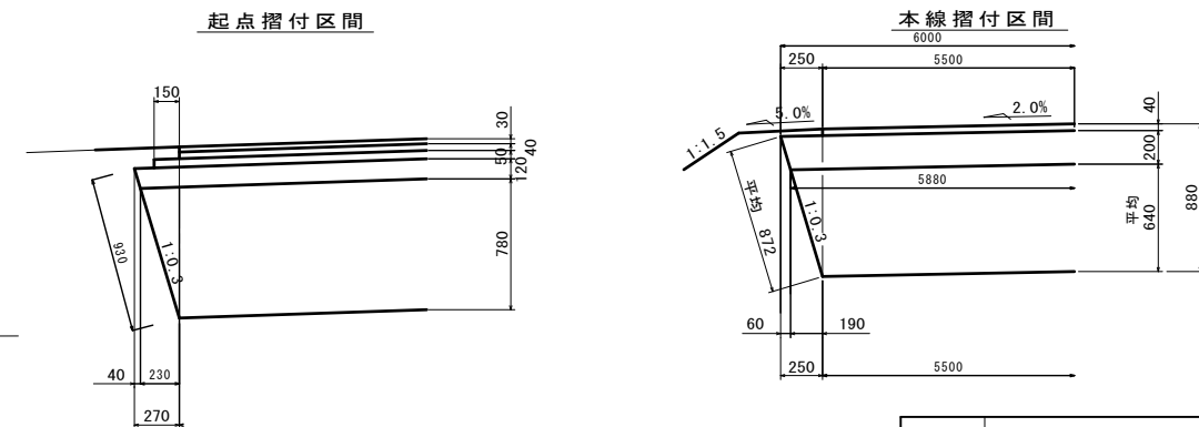
路肩詳細図 S=1:25
