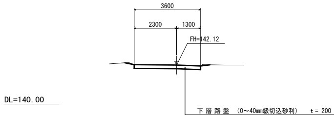
C-C断面図 S=1:100
