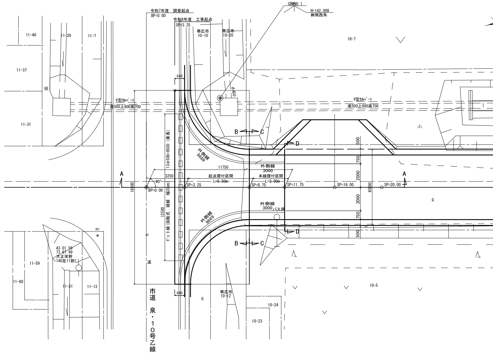
平面図 S=1:100
