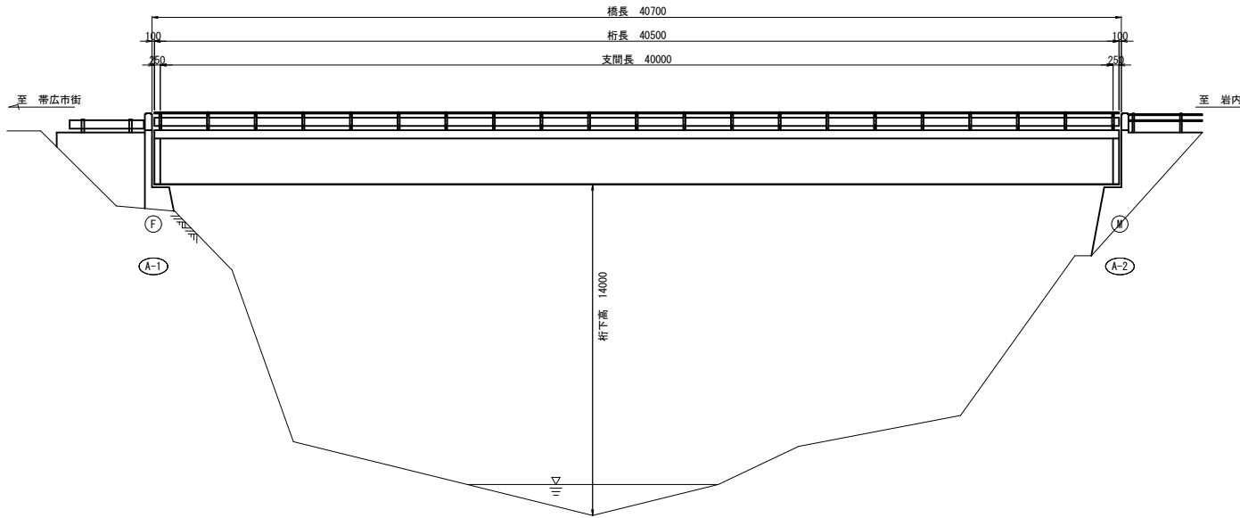
側面図 S=1:100
