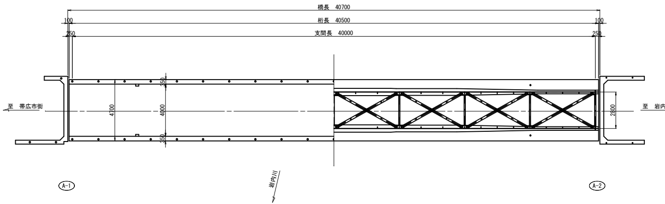
平面図 S=1:100
