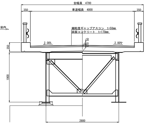
現況橋梁緒元
