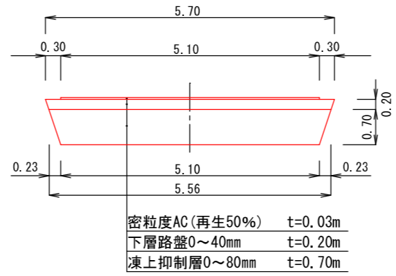
土工定規図 ② 1 : 100
