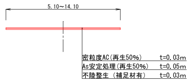
土工定規図 ① 1 : 100
