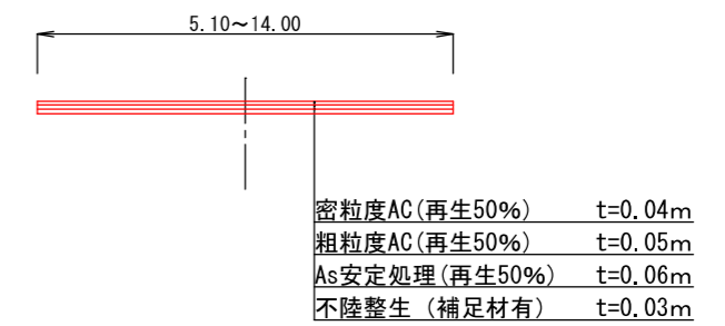
土工定規図 ③ 1 : 100
