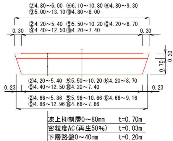
土工定規図 ②⑤⑥⑨⑩
