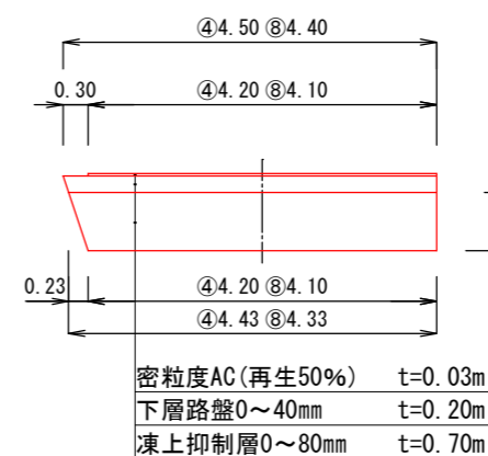
土工定規図 ④⑧
