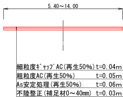
土工定規図 ①
