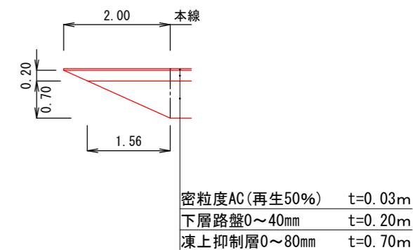
摺付部断面図
