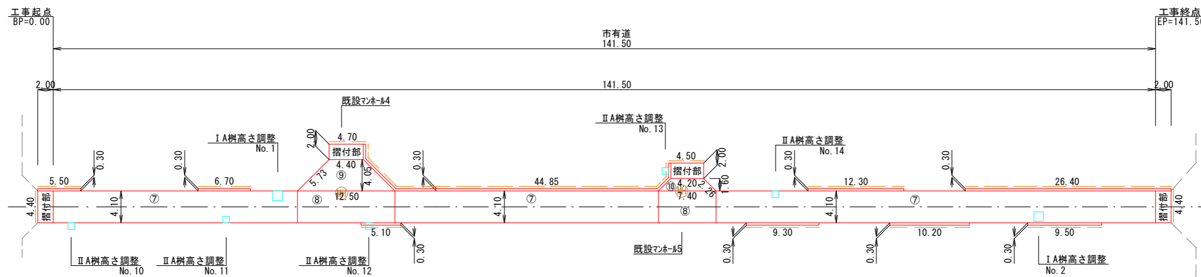
土工定規図 ①
