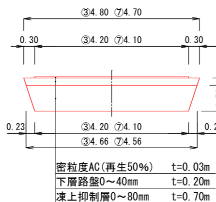
土工定規図 ③⑦
