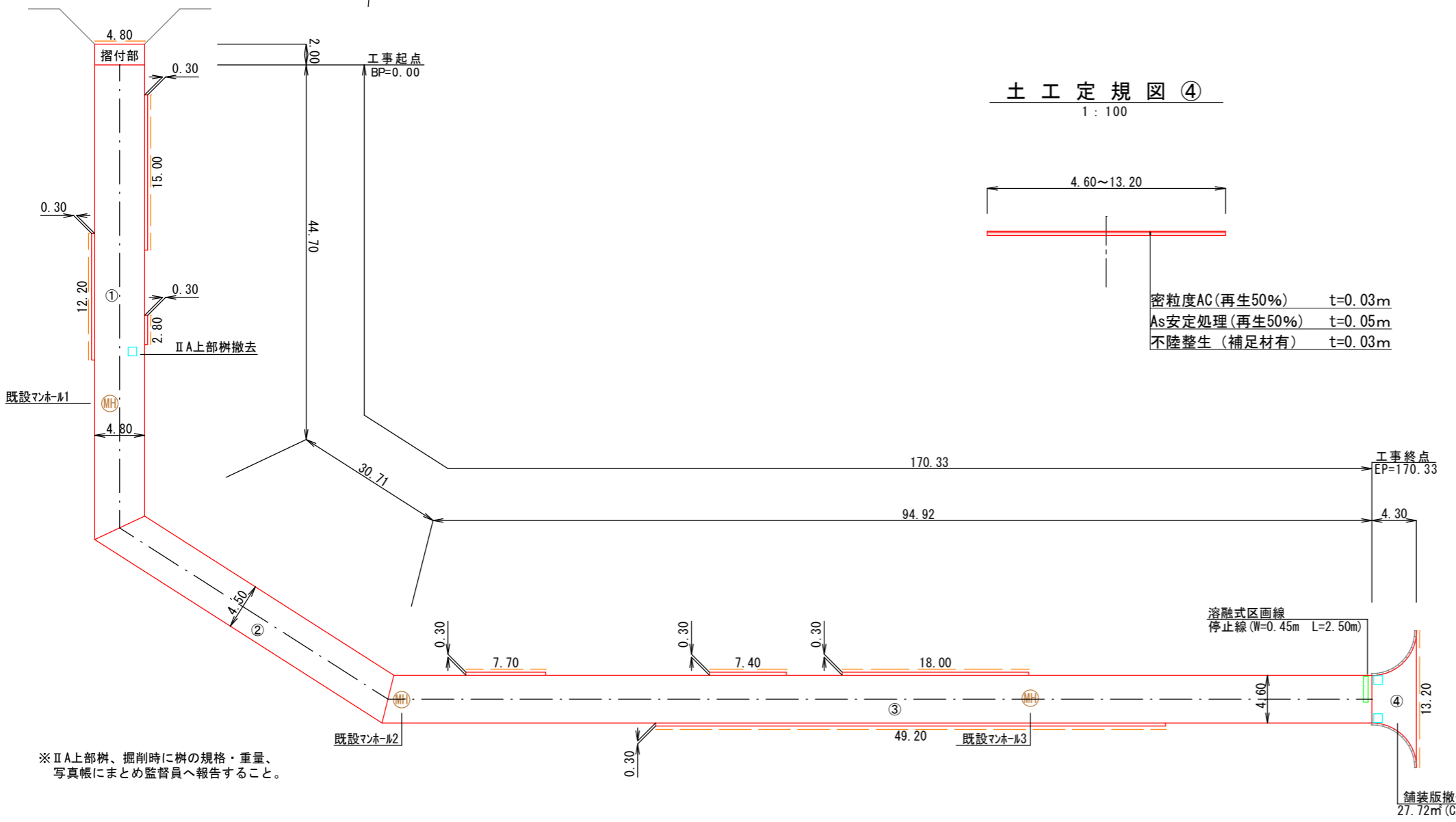
現況平面図 1:500 (帯広市東11条南5丁目)
