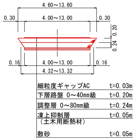
土工定規図②③ 1 : 100
