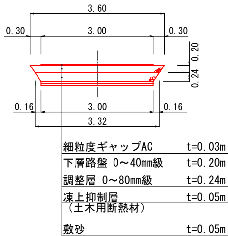
土工定規図① 1 : 100
