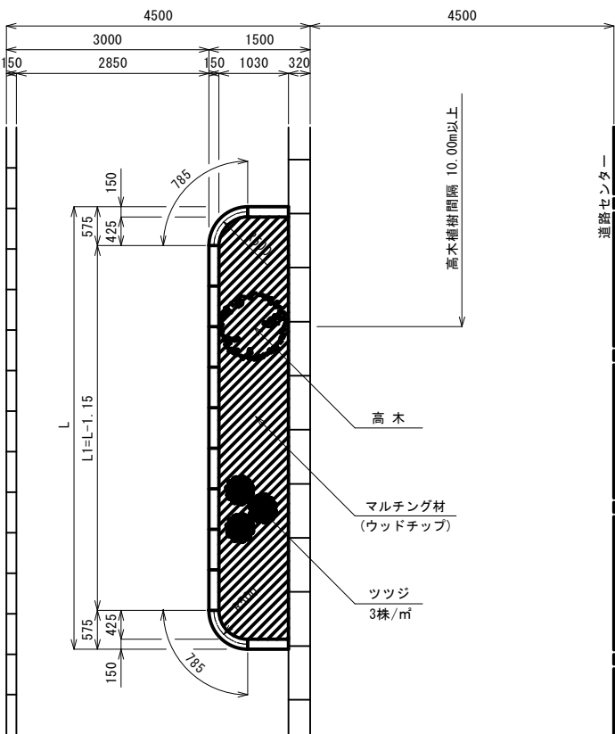
平面图 S=1:50
