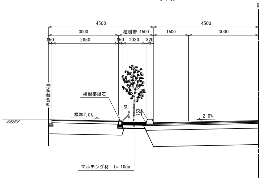
側 面 図 S=1:50
