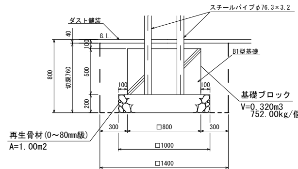
参考図
