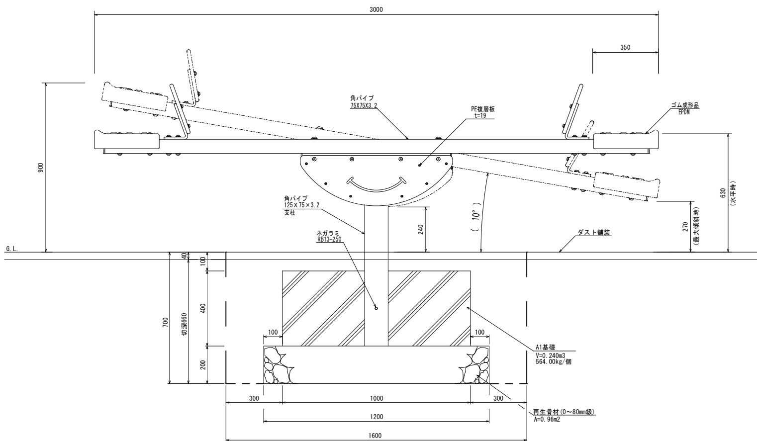
側面図
