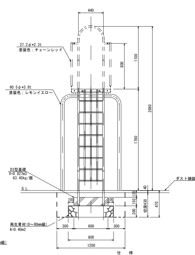
正面図
