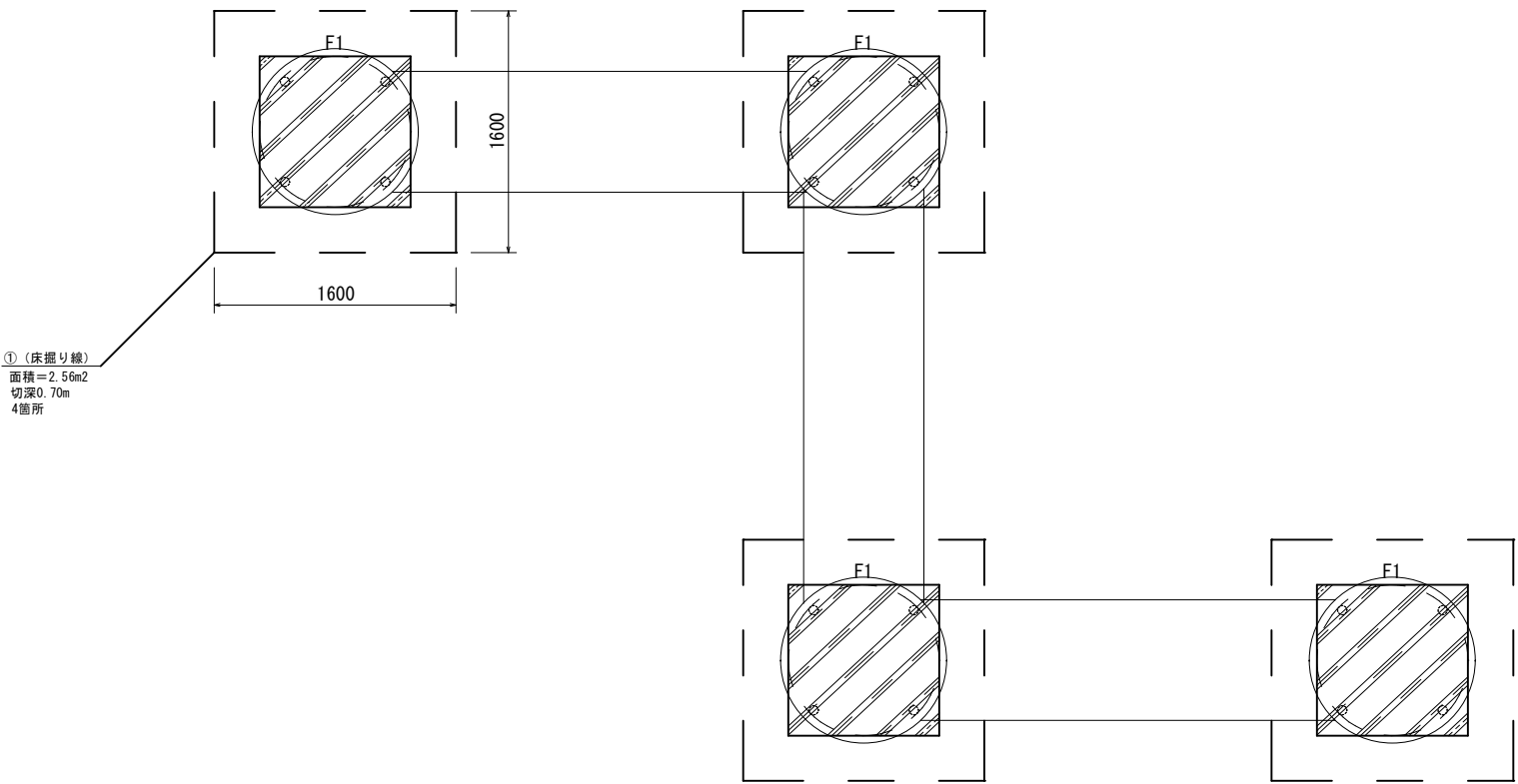
平面図 S=1:25
