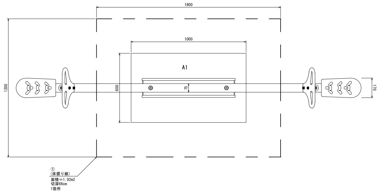
平面図
