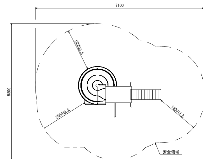
安全領域図
