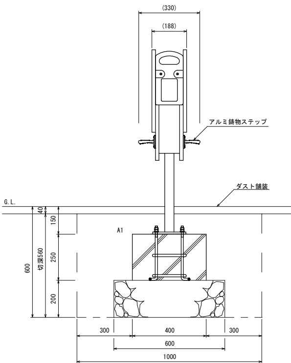
立面図
