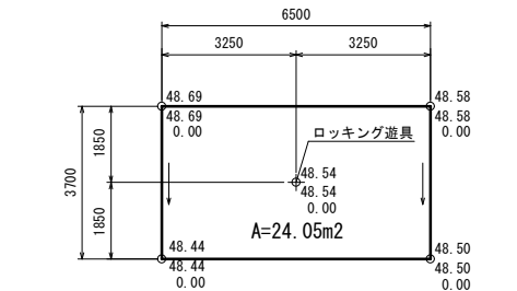
ダスト舗装詳細図 S=1/100
