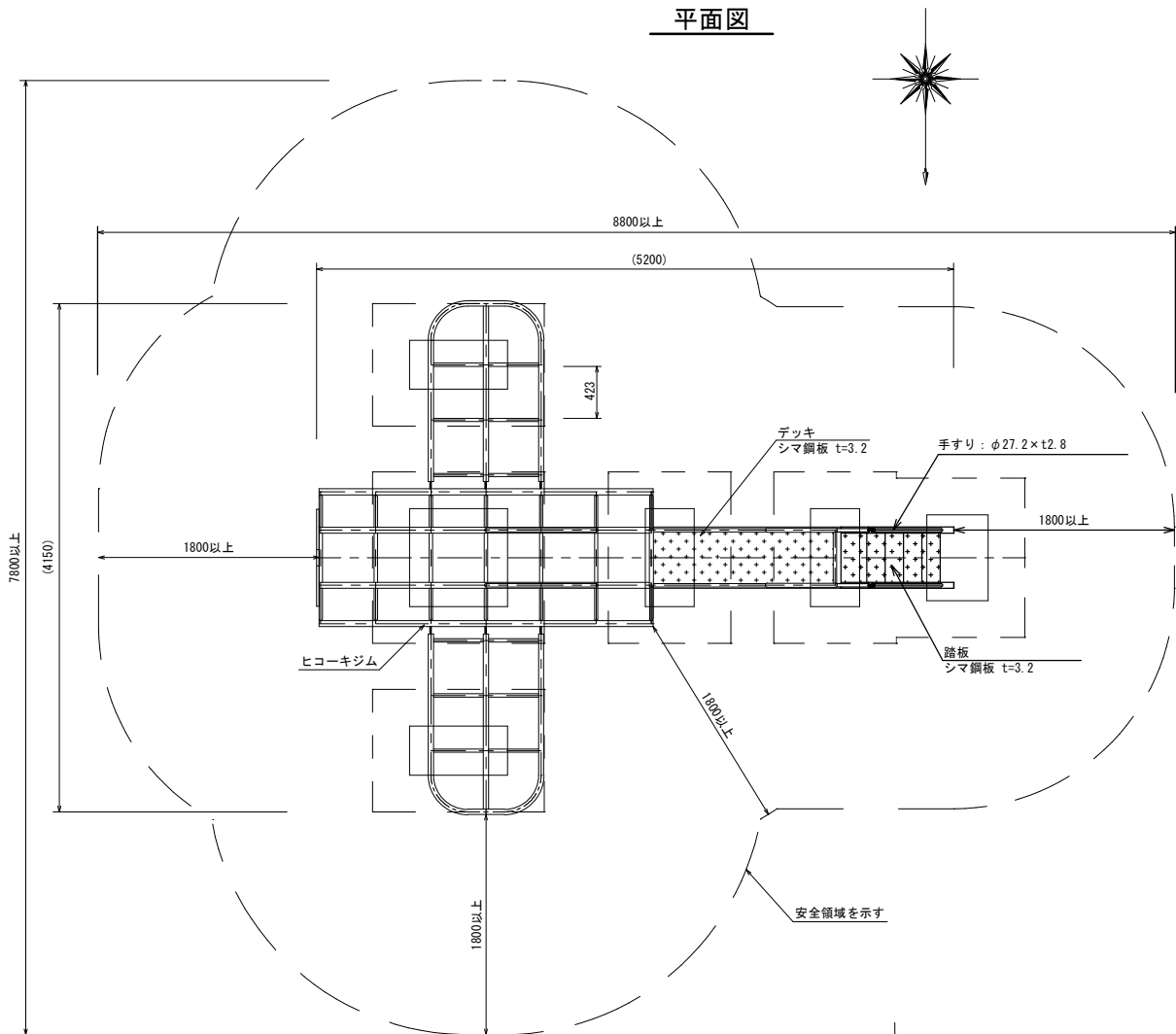
平面図
