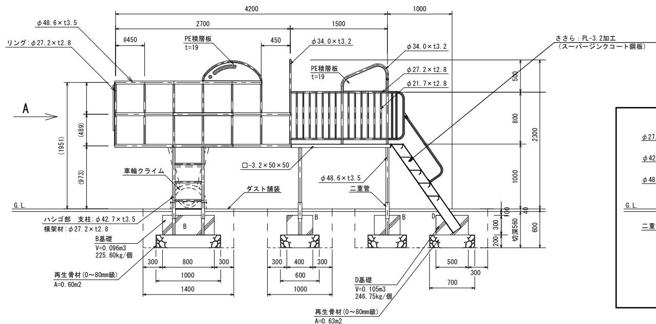
立面図
