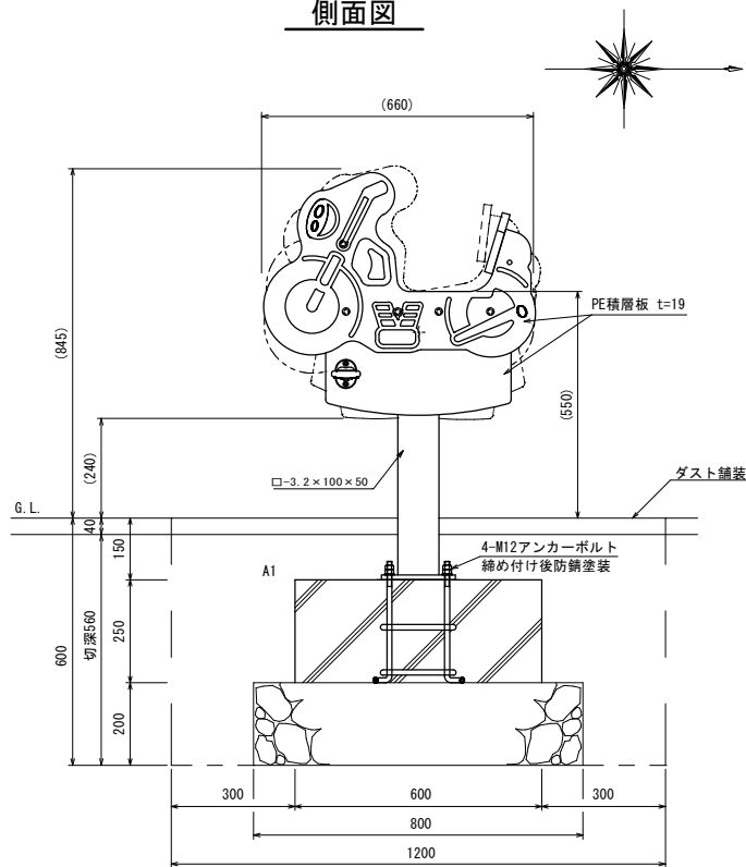
参考図
