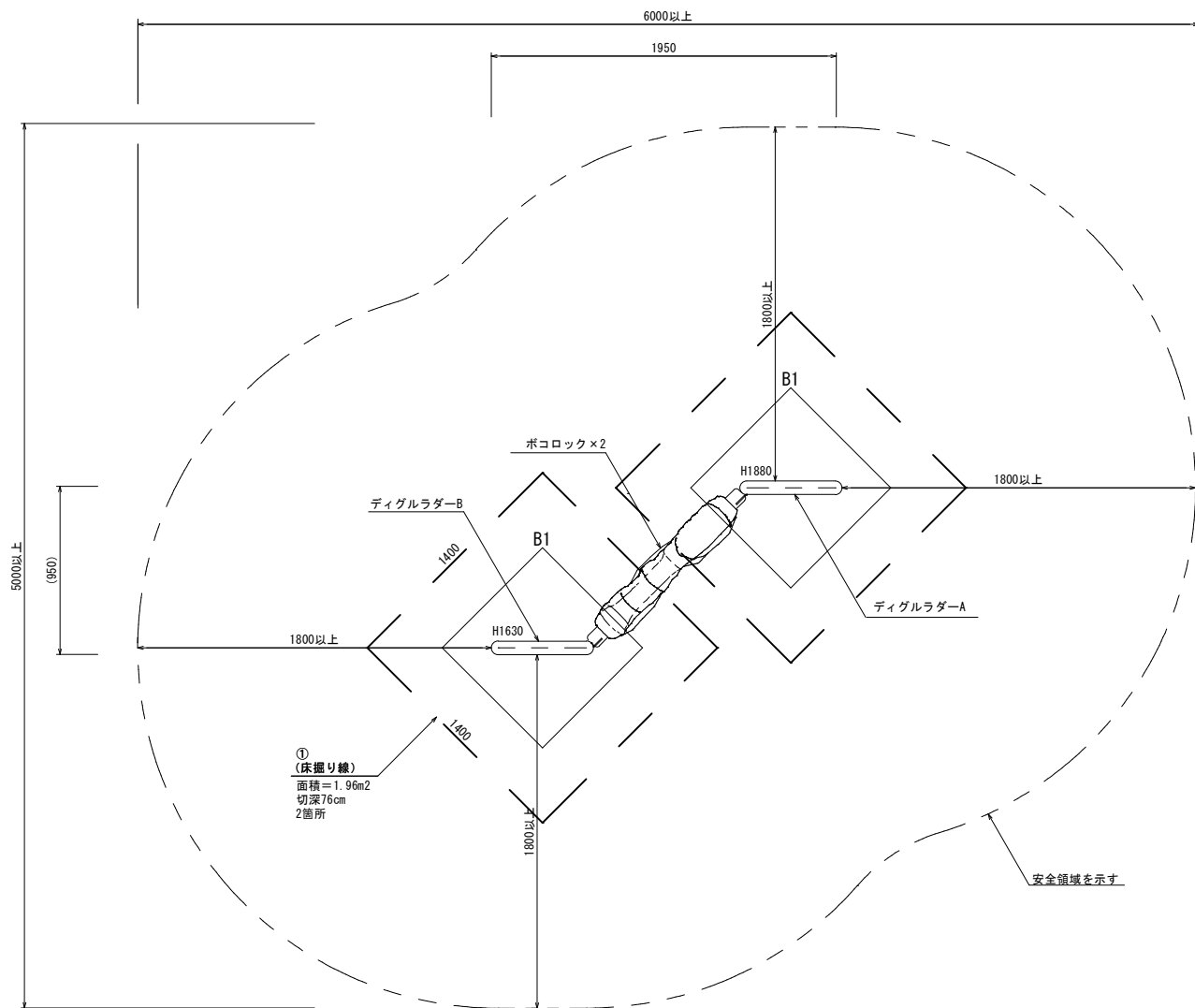
平面図
