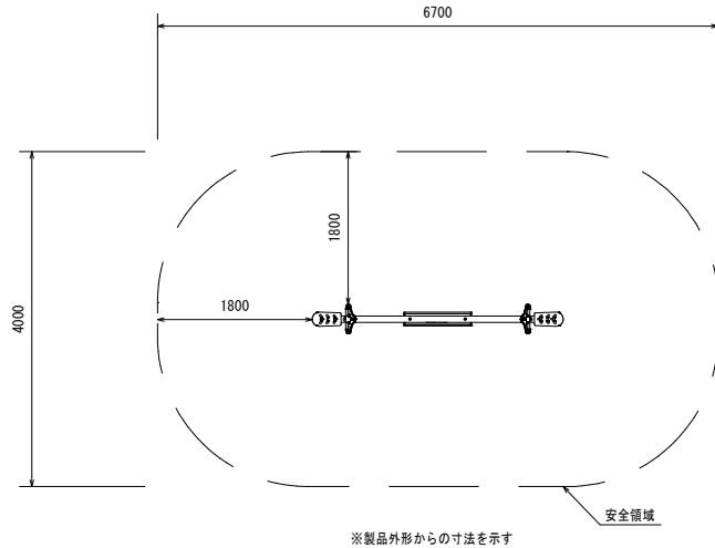
安全領域図
