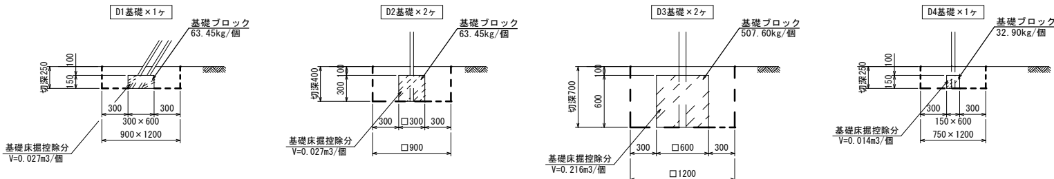
正面図
