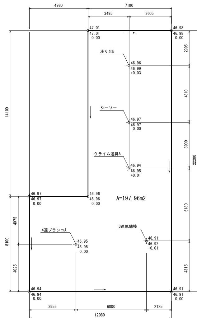
ダスト舗装詳細図 S=1/100
