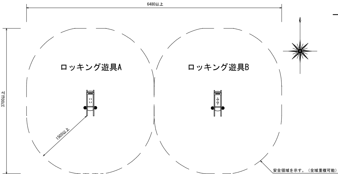
安全領域図 S=1/30
