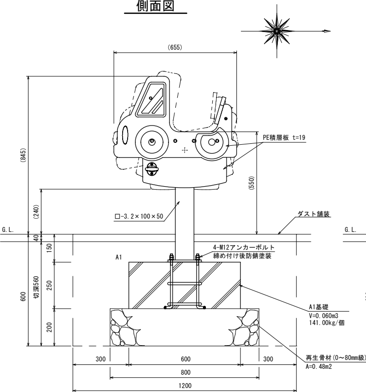
側面図
