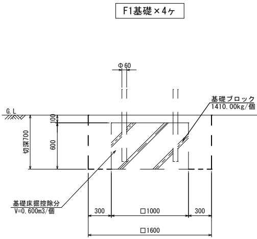
正面図 S=1:25
