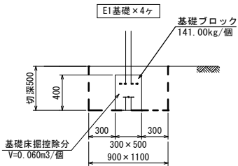
正面図
