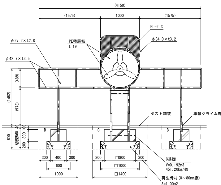
参考図
