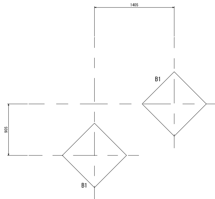
基礎伏図
