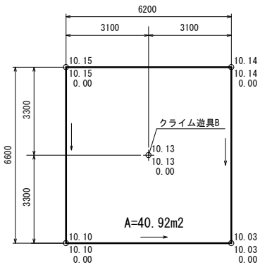
ダスト舗装詳細図 S=1/100
