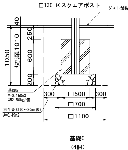
基礎詳細図 S=1/20
