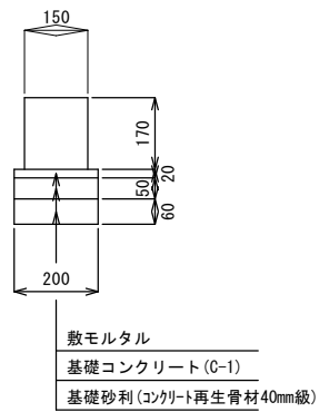
植樹帶縁石詳細図
