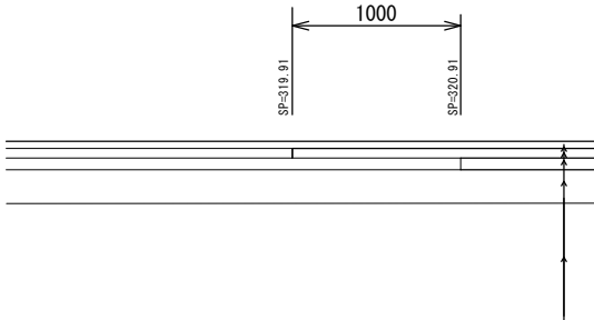
基層・上層路盤起点詳細図
