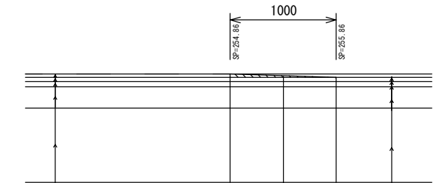
起点摺付詳細図
