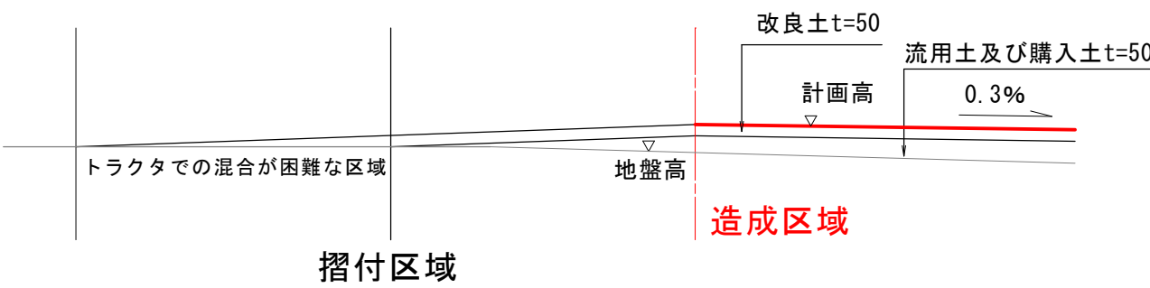
グランド'摺り付け区域標準断面図 1:30
