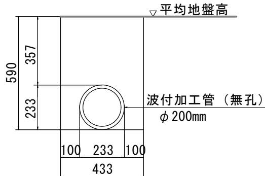
連絡渠標準断面図
