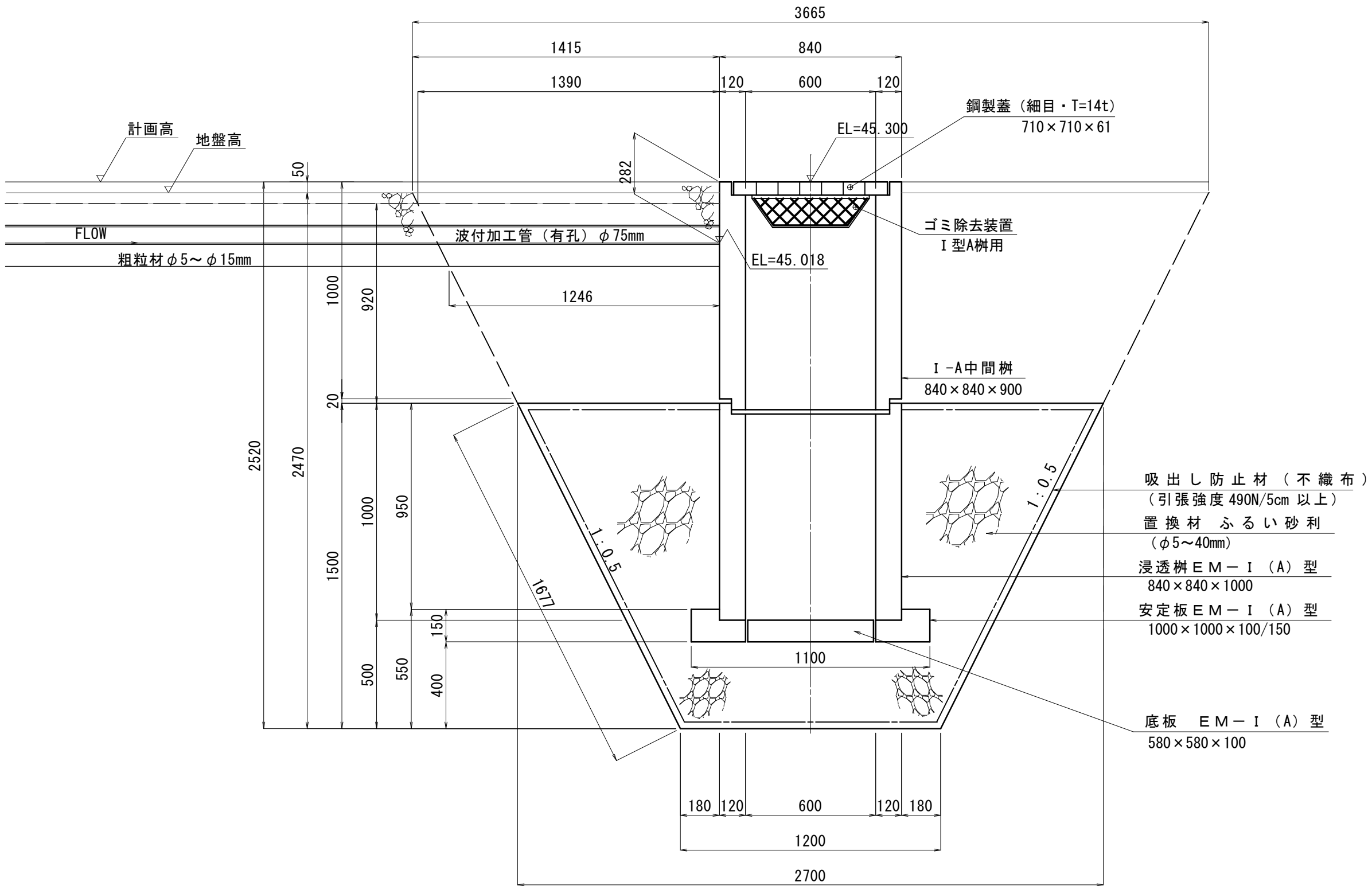
側面図
