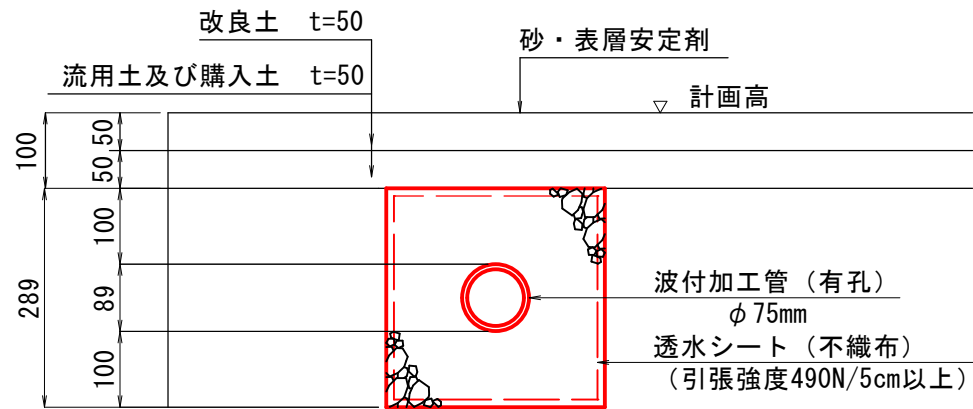
グランド'造成区域標準断面図 1:10
