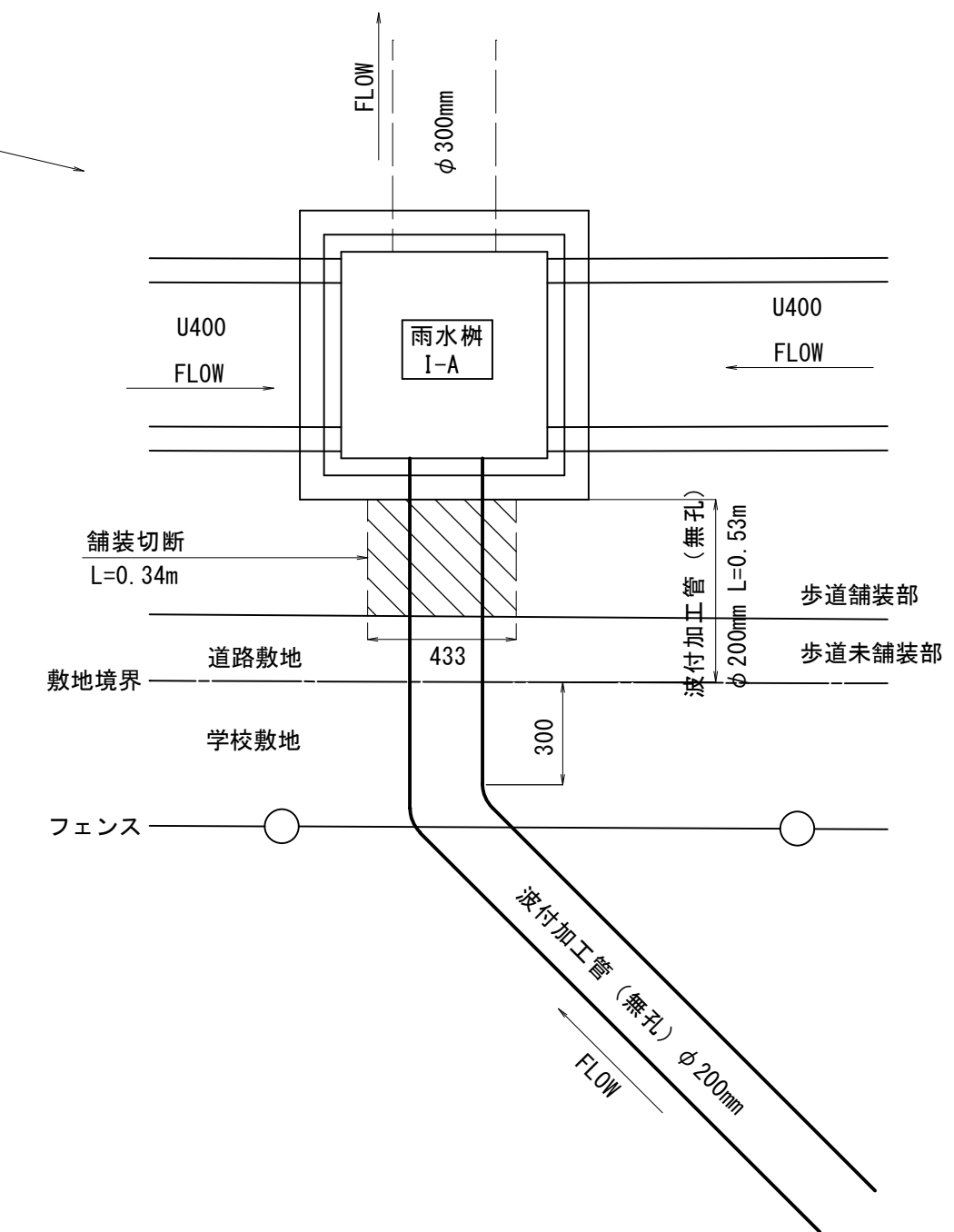
拡大図
