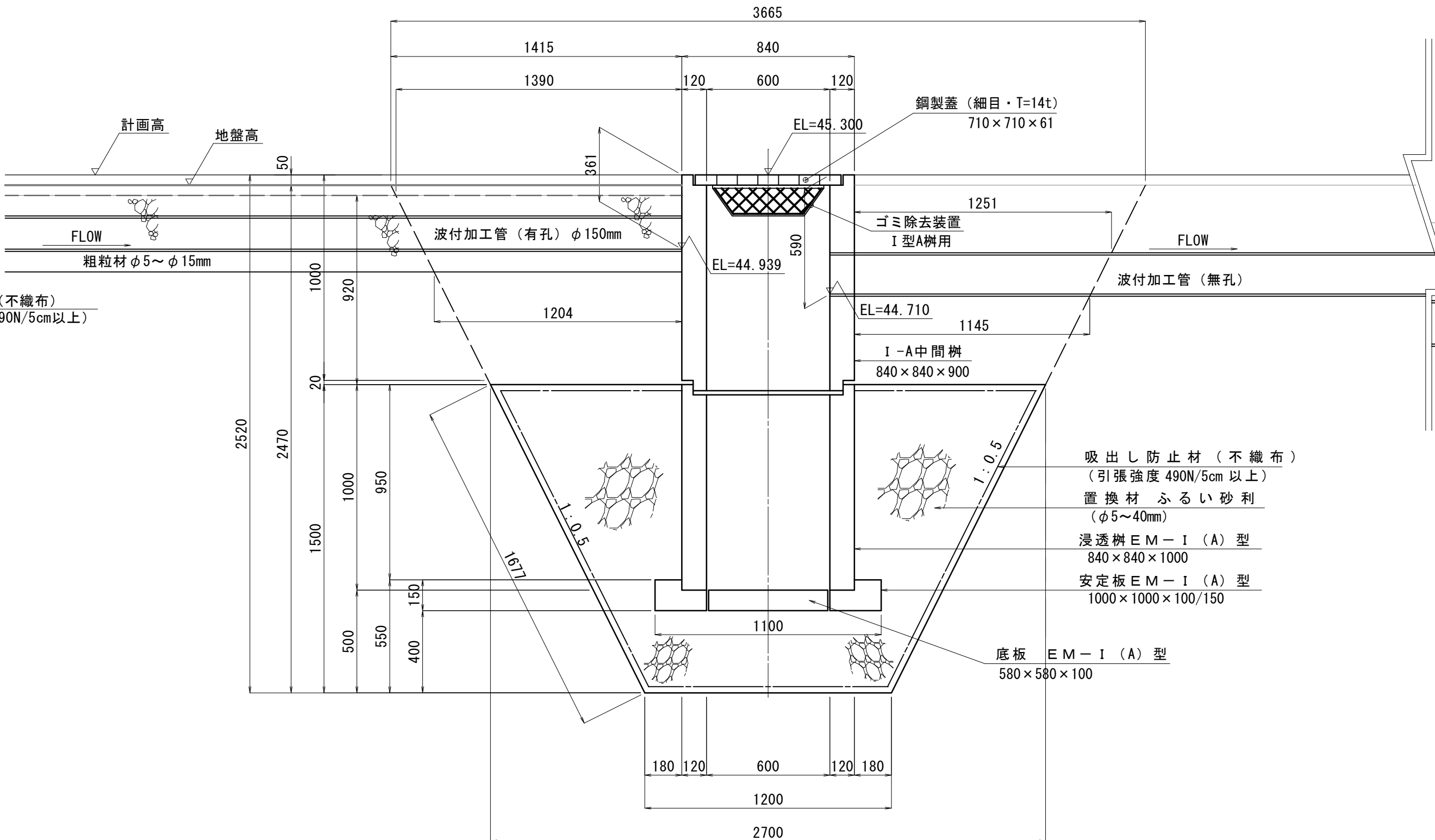
側面図
