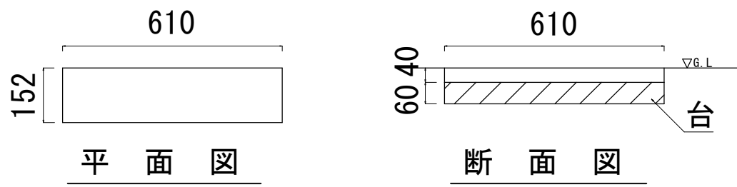
ピッチャープレート詳細図
