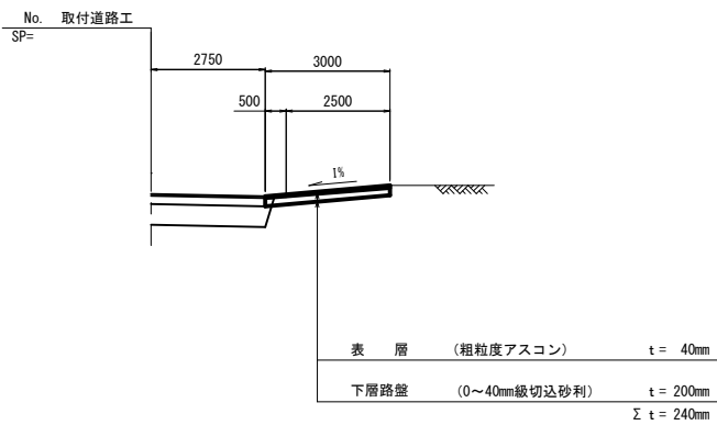
一般切土部
