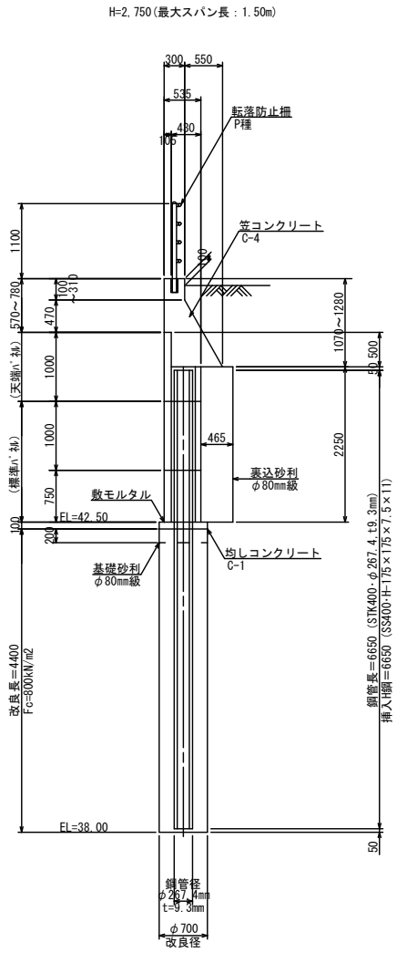
標準断面図
