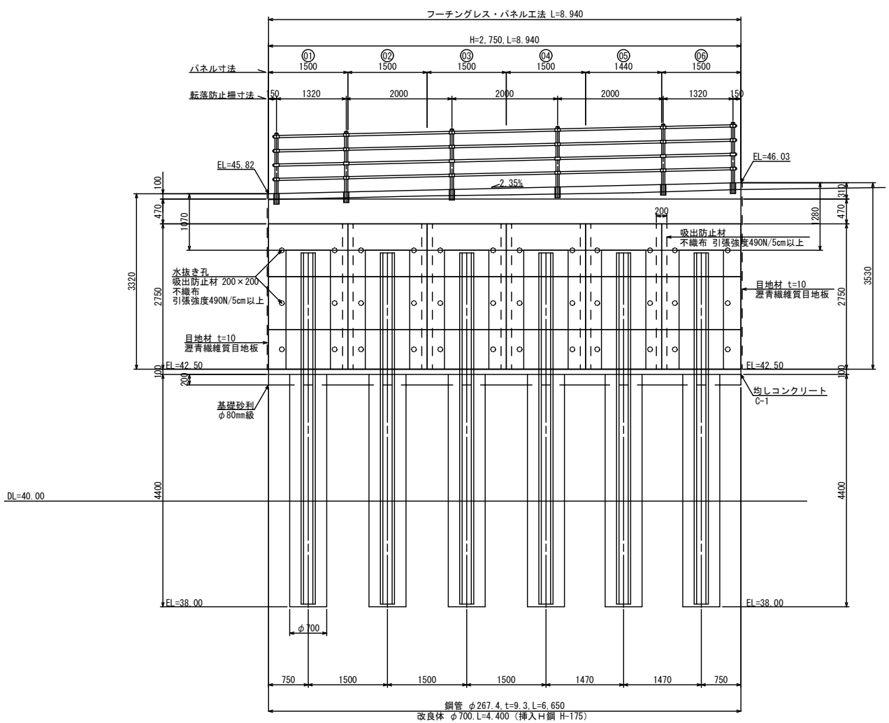
背面展開図
