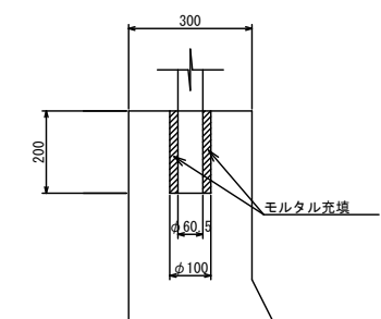
転落防止柵 支柱根入れ部
