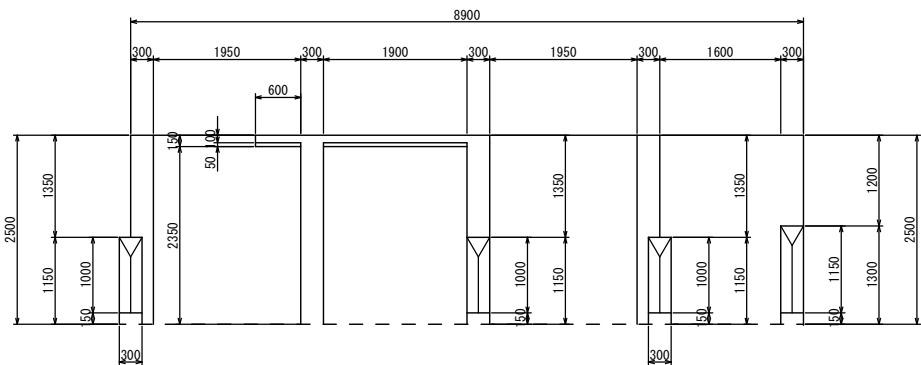
I-I
