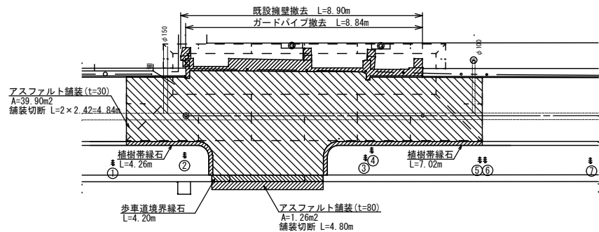
撤去平面図
