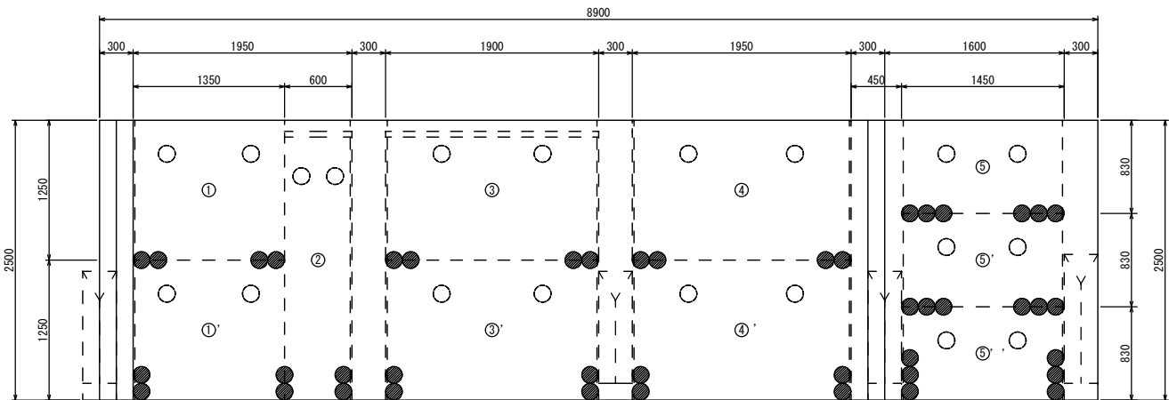
正面図
