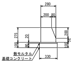
歩車道境界縁石
