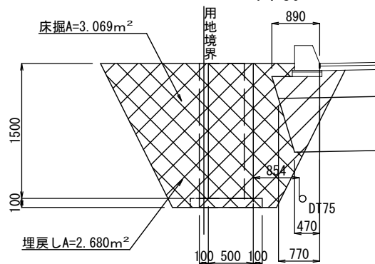
断面図(A-A') 1:30
