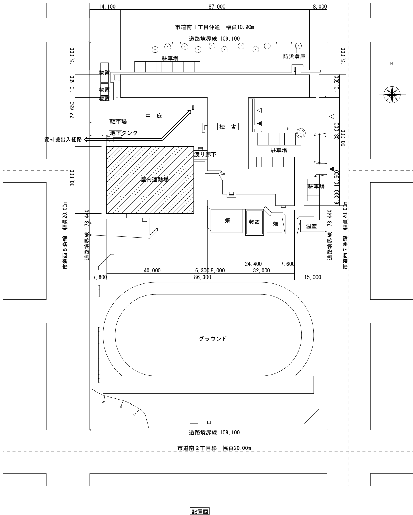
配置図
