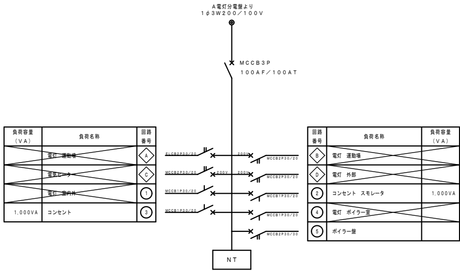
既設電灯分電盤（体育館分電盤） ※停電時は、×印のブレーカーを開放する。
