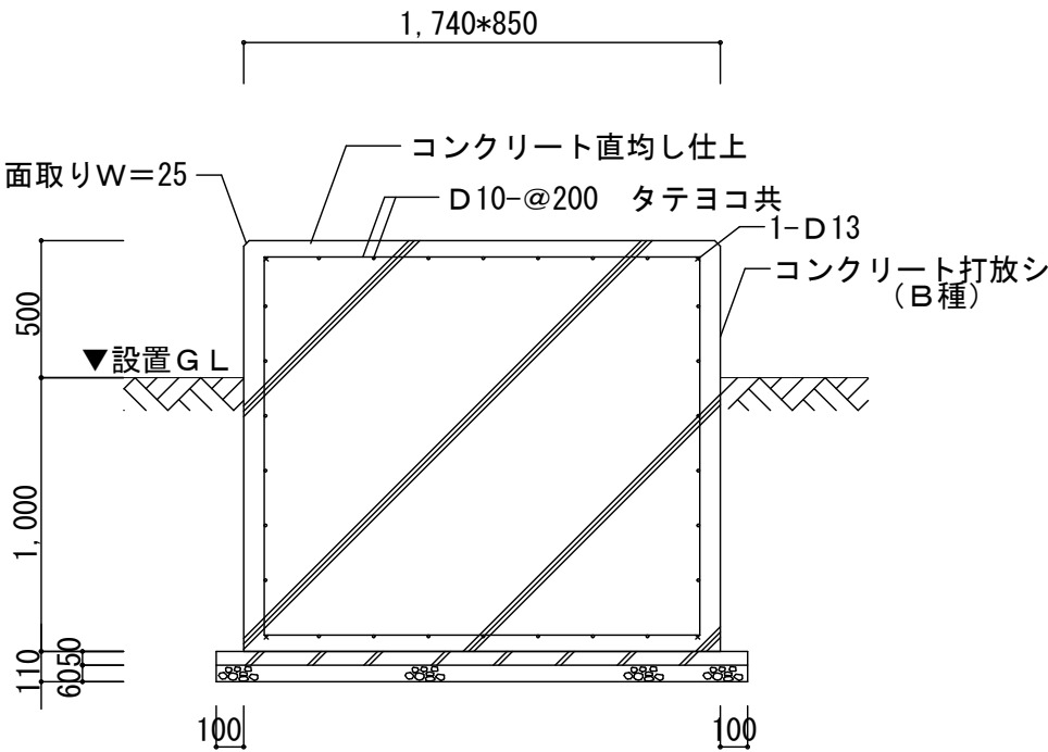
断面図
