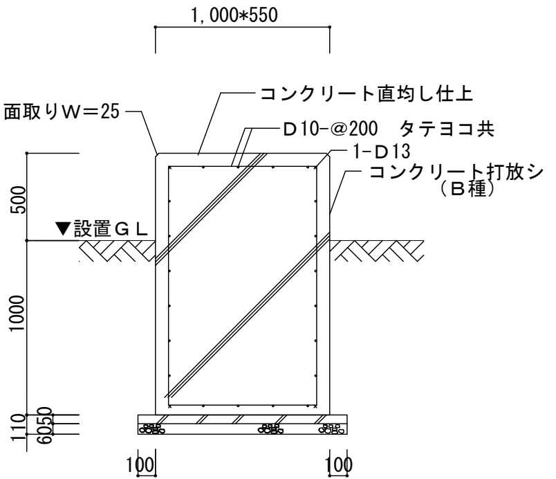
断面図
