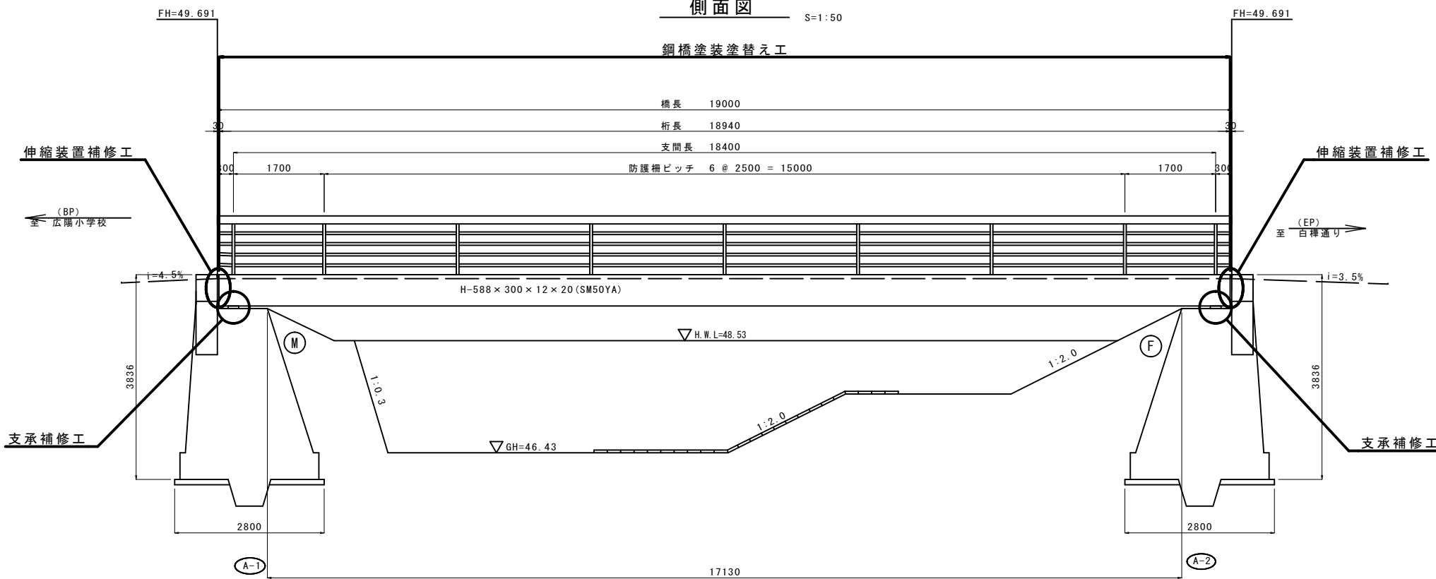
側面図
