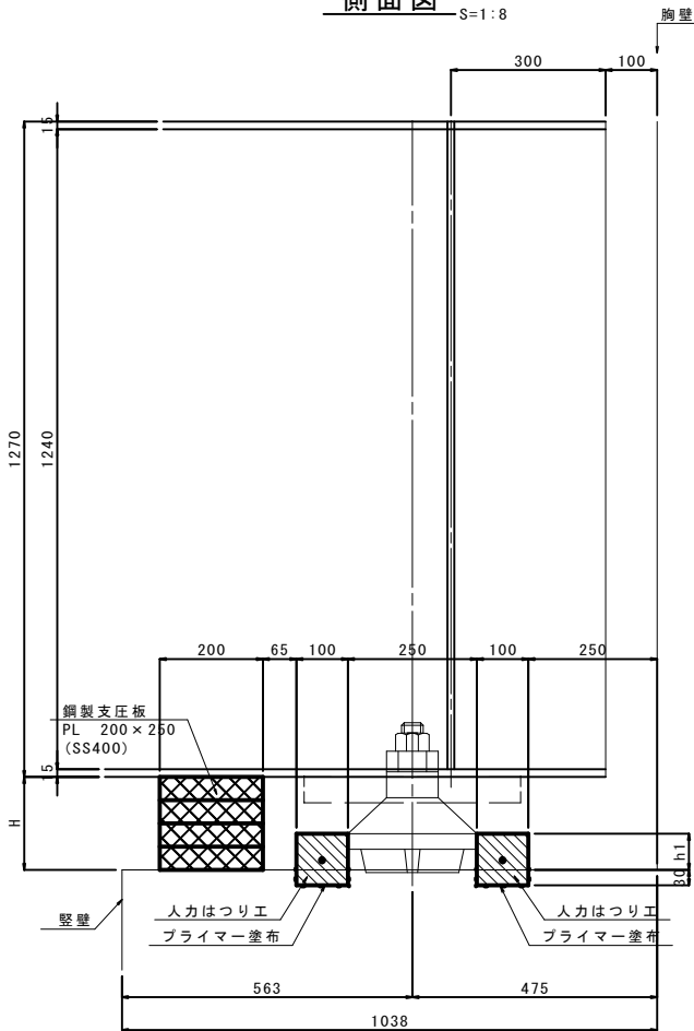
側面図
