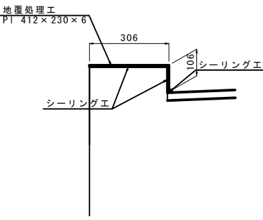
橋台部断面図
