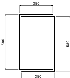
鉄筋加工表
