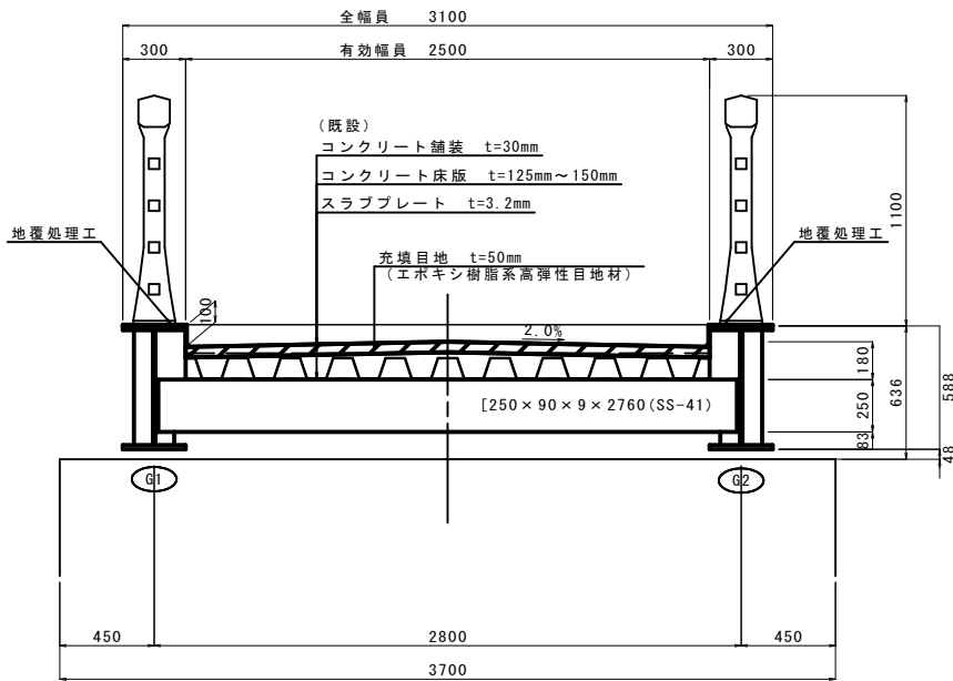
上部工断面図
