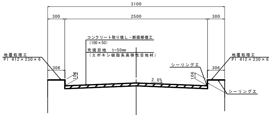
上部工断面図
