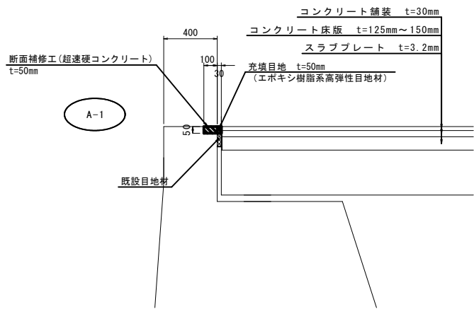
断面図
