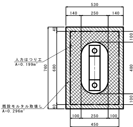
施工平面図
