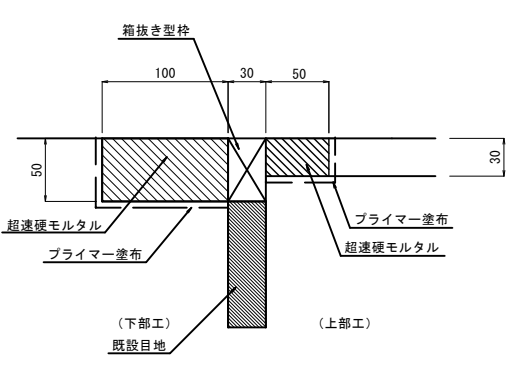
②箱抜き型枠及び断面修復工
