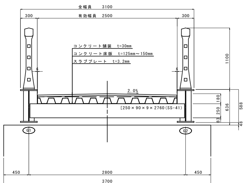
プランクシート詳細図
