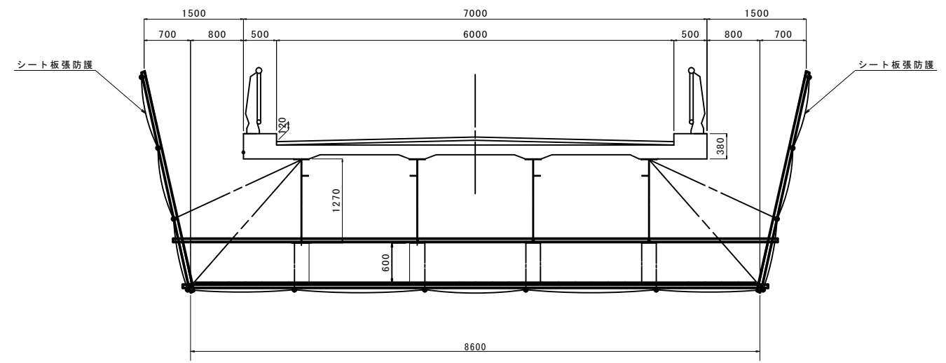
断面図 (A-A) S=1:40
