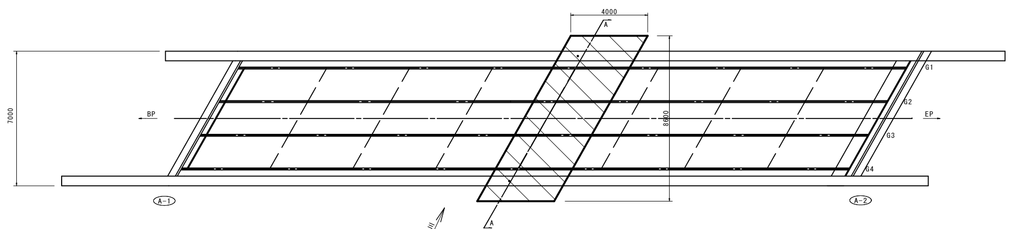
断面図 (A-A) S=1:40
