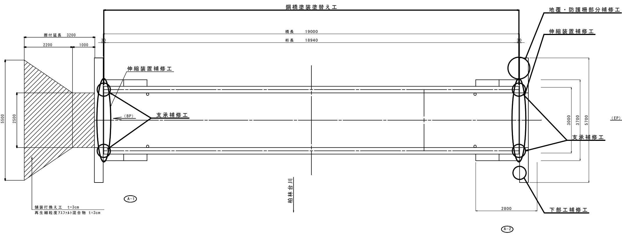
平面図
