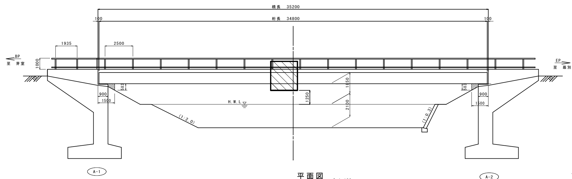
側面図 S=1:100
