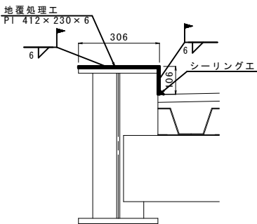
橋梁部断面図
