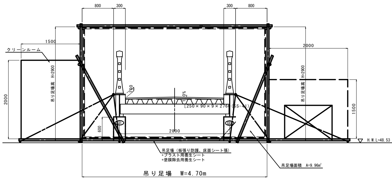
断面図
