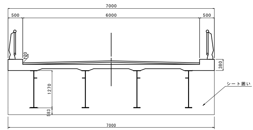
断面図 (橋台部共通) S=1:40
