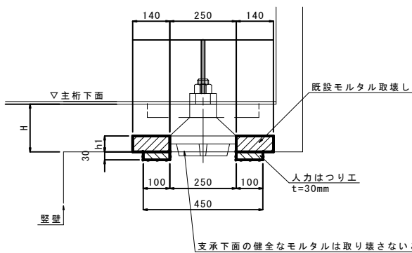
施工断面図
