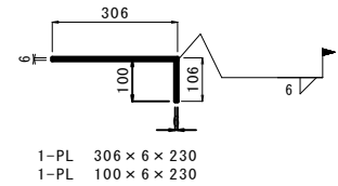
地覆処理プレート詳細図
