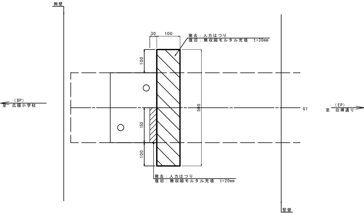
平面图 S=1:5
