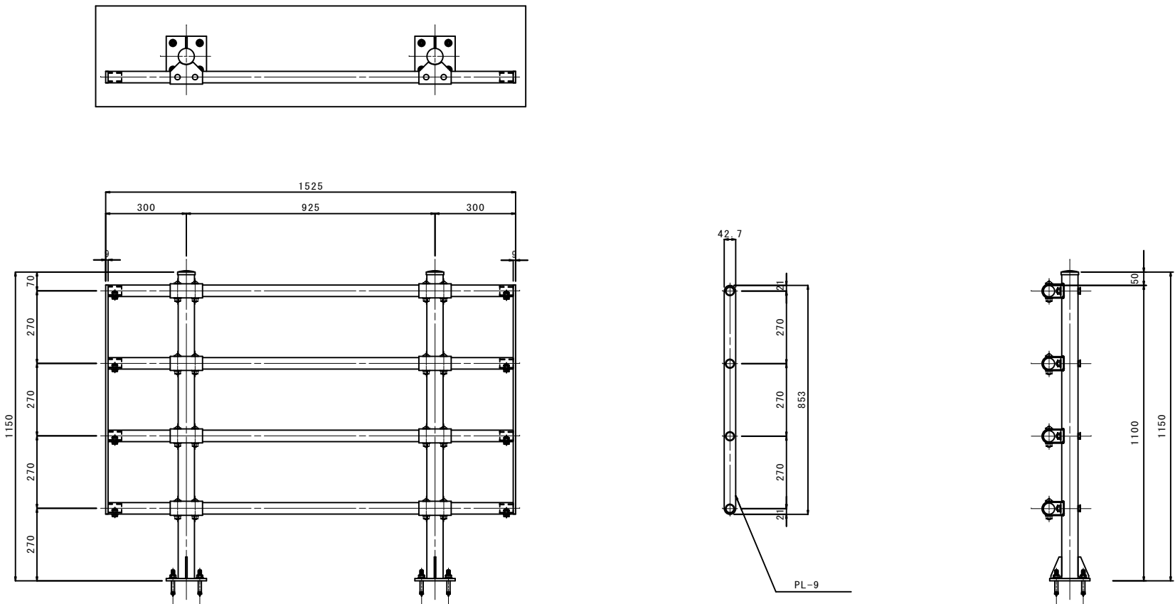
転落防止柵詳細図
