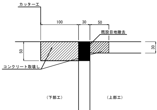
①既設目地撤去およびコンクリートの取壊し
