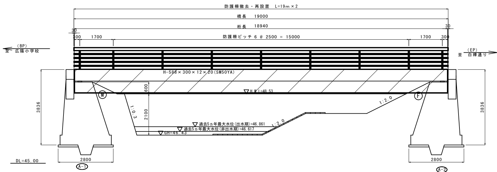
側面図
