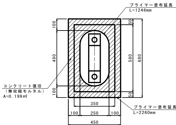
施工平面図
