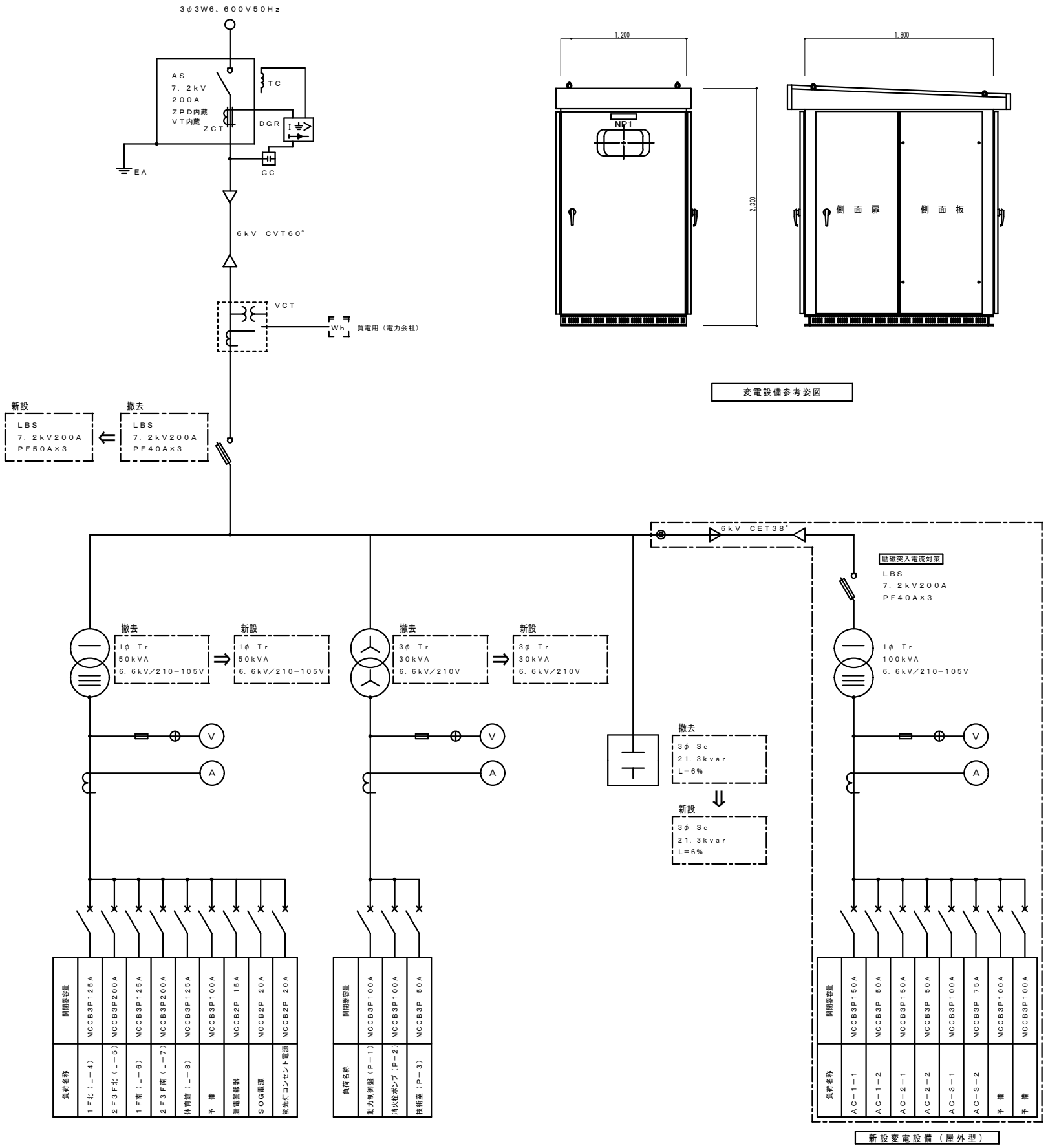
改修後単線結線図
