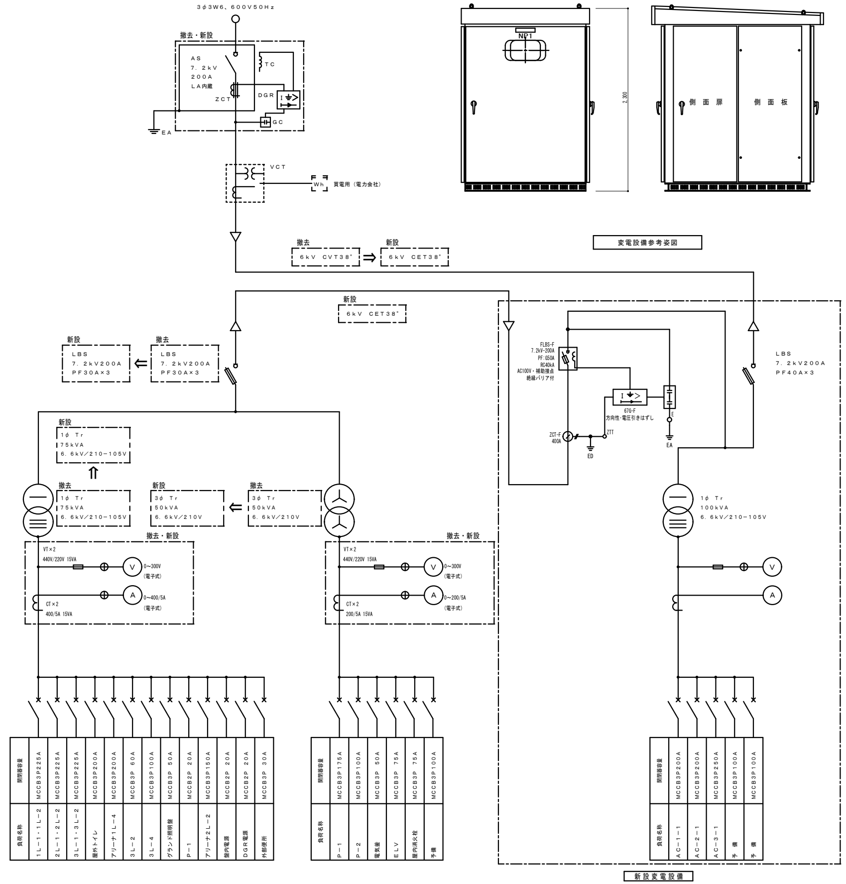
改修後単線結線図
