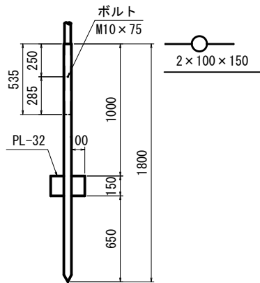
基礎管 S=1:20
