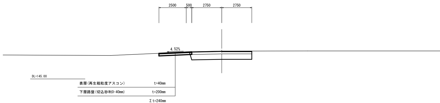
No. 14 取付道路工 (L) SP=555.50
