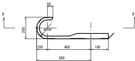
袖ビーム S=1:10
