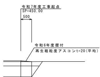
起点部撤去図
