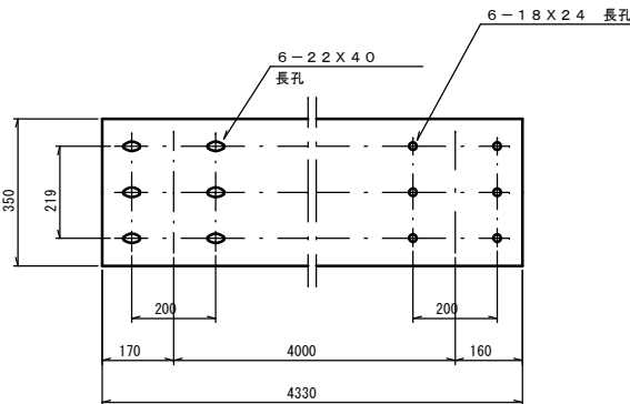
ビーム S=1:10
