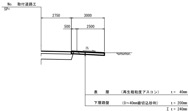
一般盛土部
