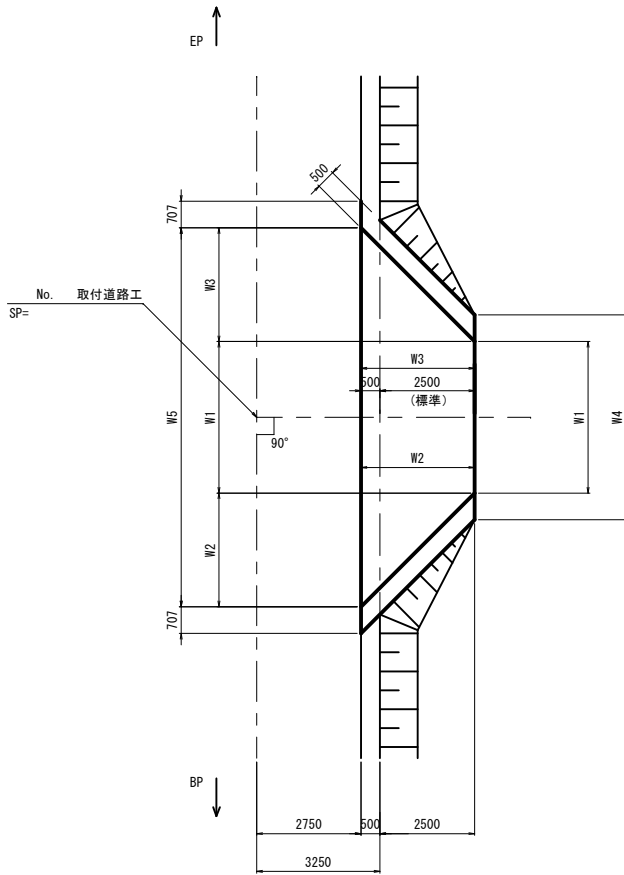
平 面 図
