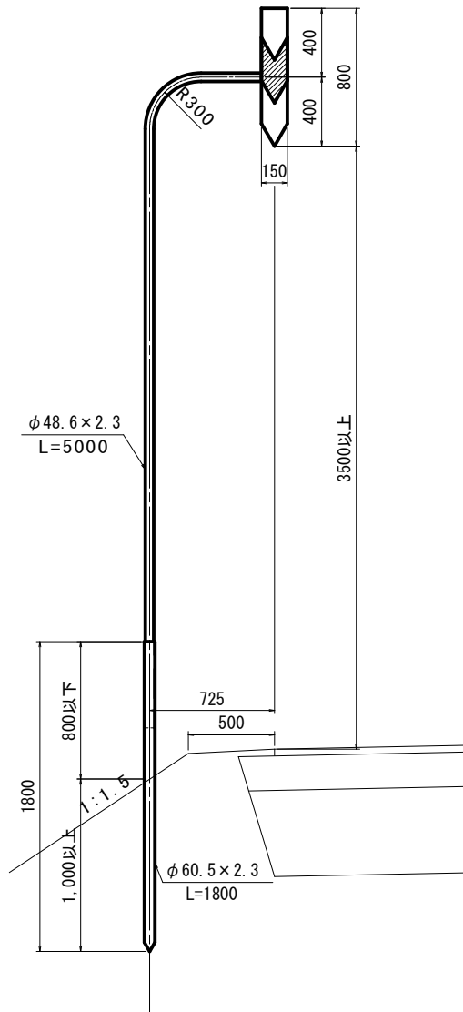
正面図 S=1:20
