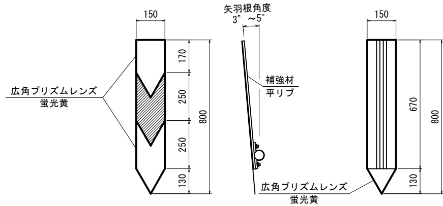
矢羽根 S=1:10
