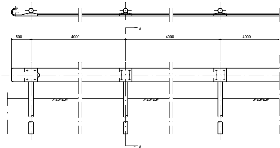
平面・立面図 S=1:30
