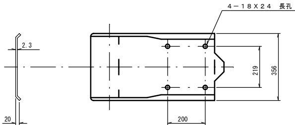
B-B断面 S=1:10
