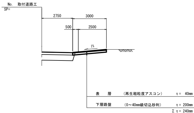
一般切土部
