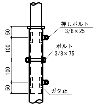
A詳細
