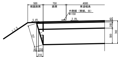
路肩詳細図 S=1:25
