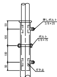
ジョイント部 S=1:5
