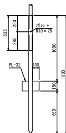
基礎管 S=1:20
