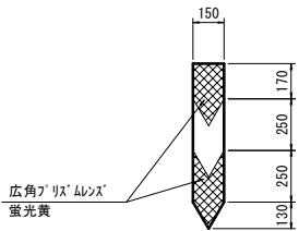
矢羽根詳細図 S=1:20
