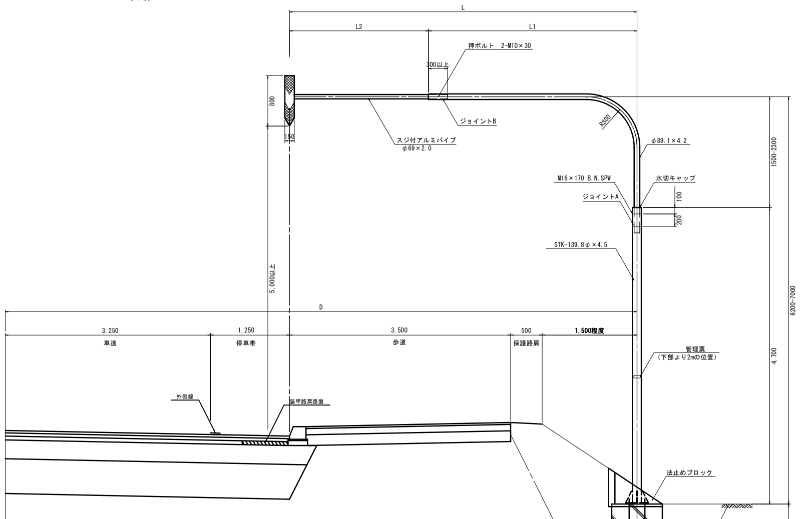
大型鋼製スノーポール S=1:30
