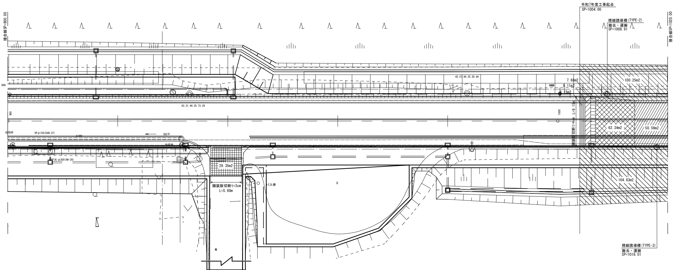
起点部撤去図 (車道)
