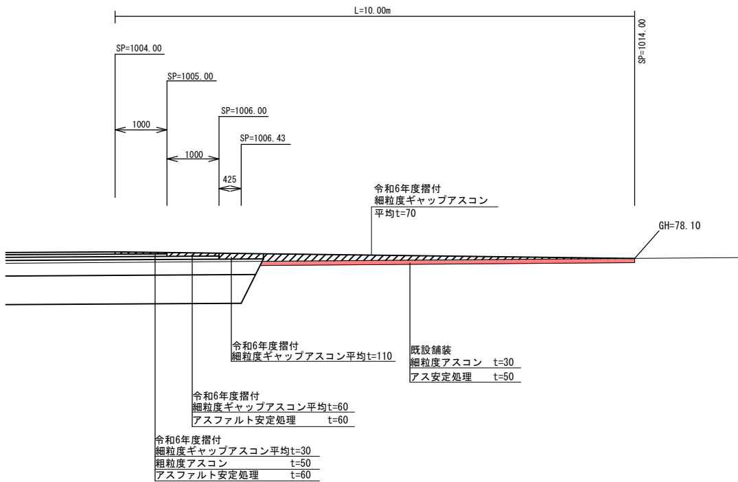
起点部撤去図 (車道)
