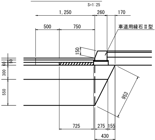
歩道(マウントアップ)
