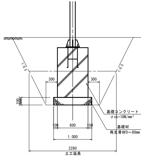
側面図
