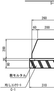
車道用縁石Ⅱ型
