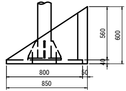
法止めブロック詳細図 S=1:20
