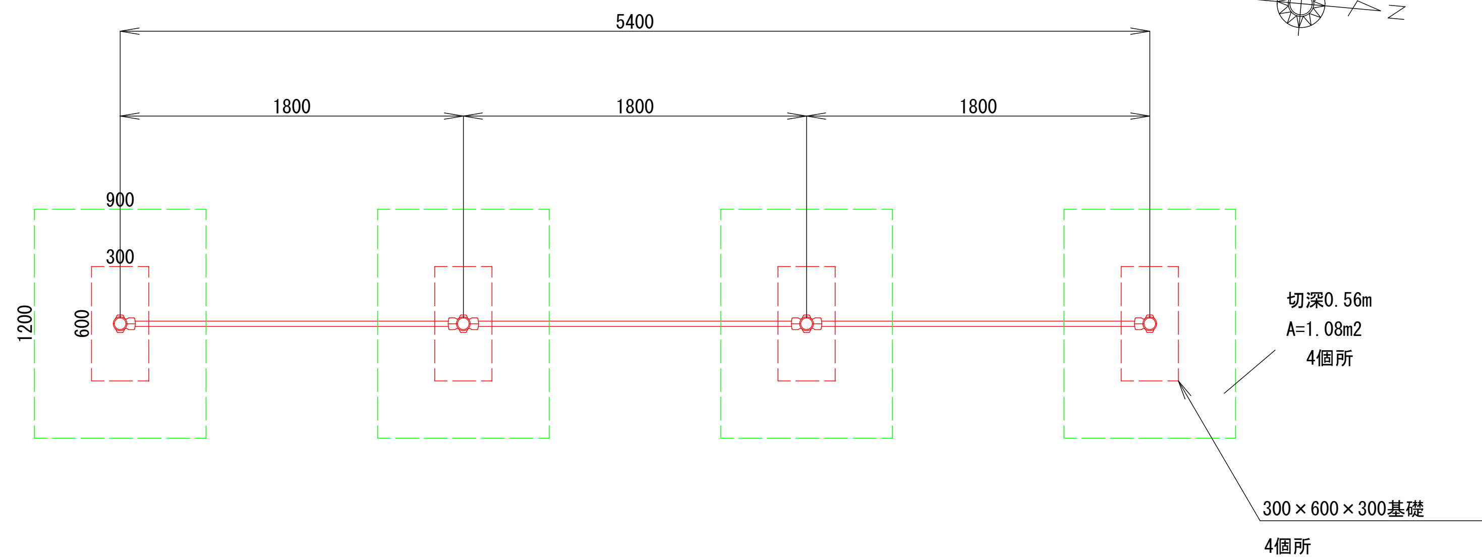
平面図 S=1/20
