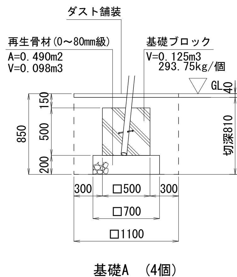
基礎詳細図 S=1:25
