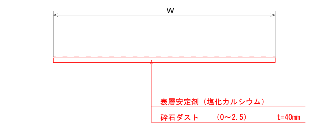
ダスト舗装詳細図
