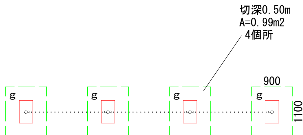
基礎平面図 1/50
