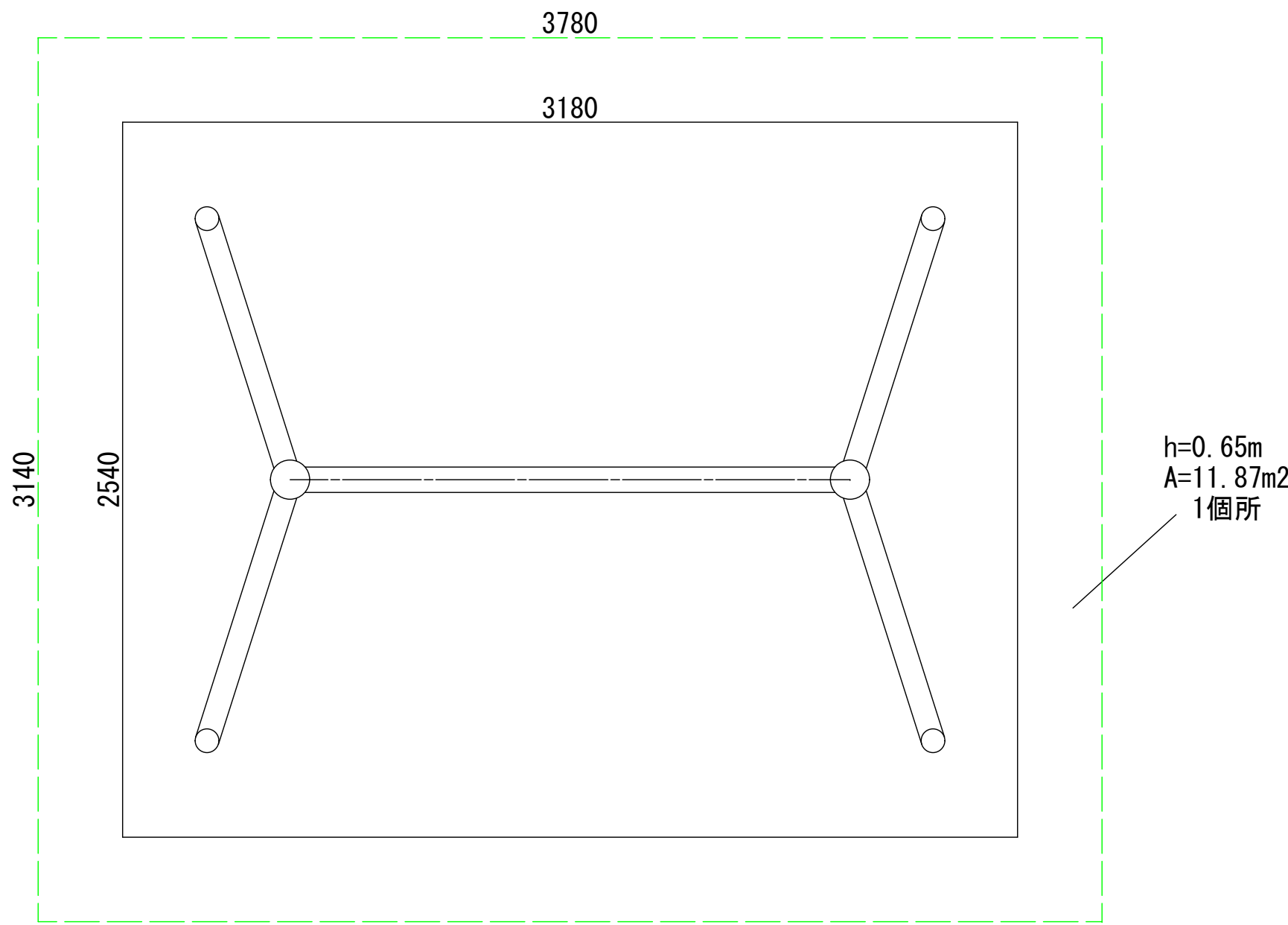
基礎平面図
