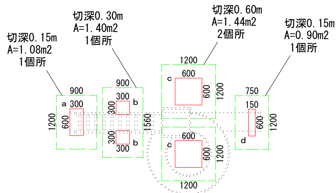
基礎平面図 1/50
