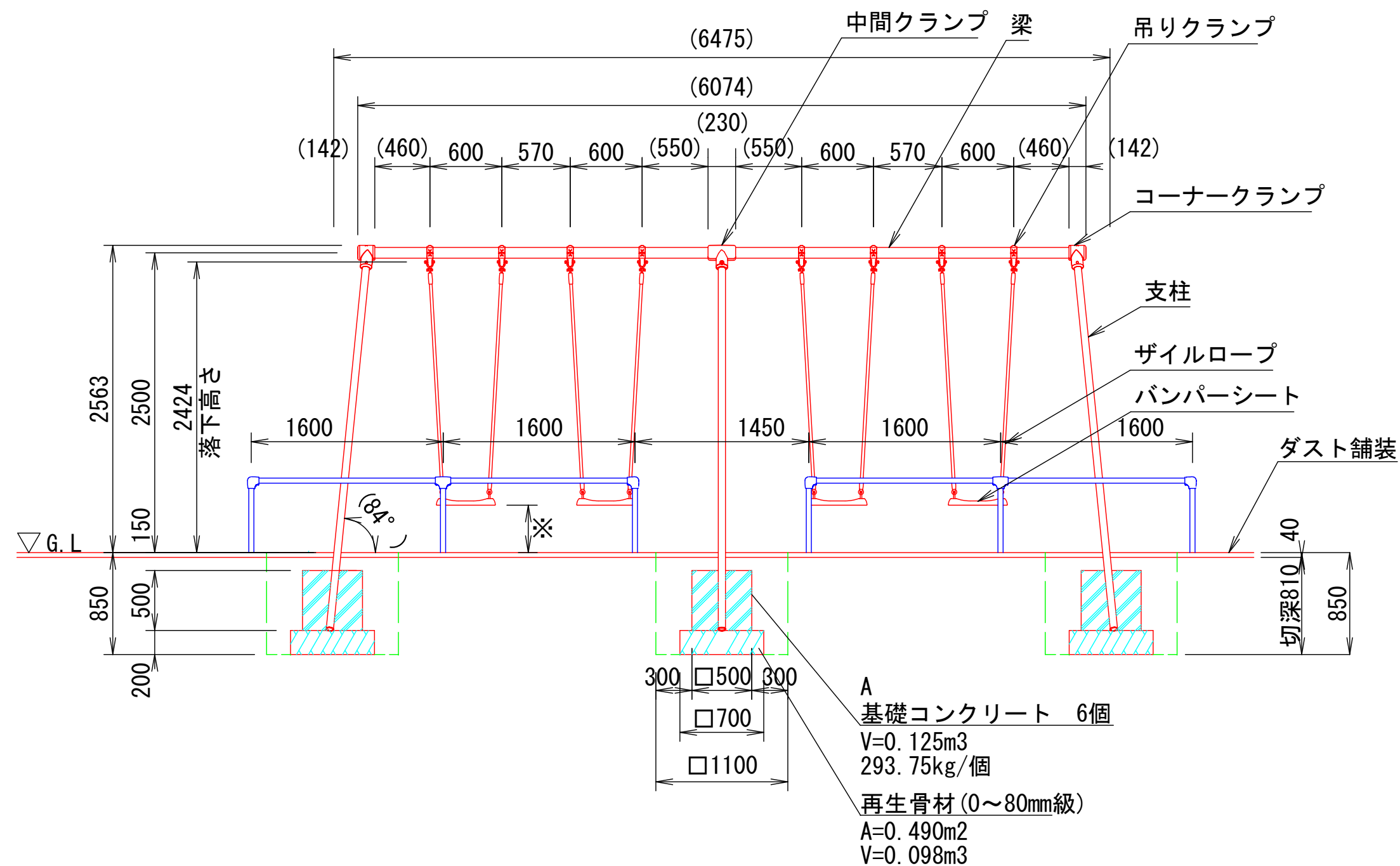
立面図 S=1/40
