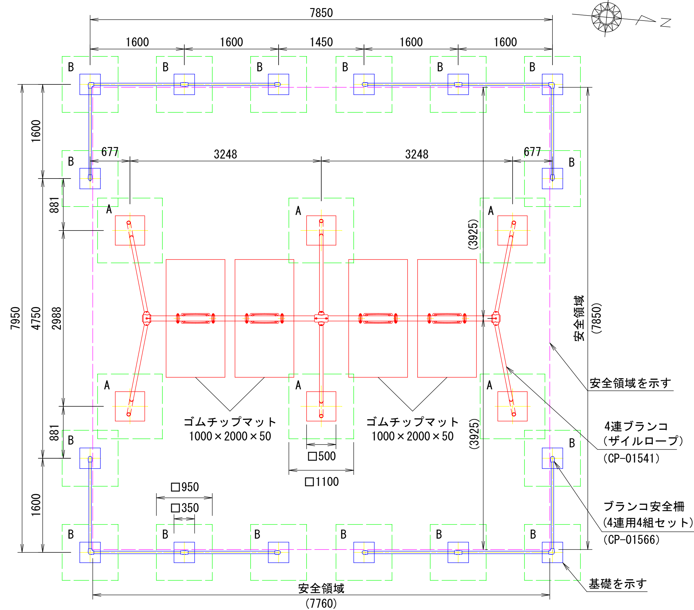
平面図 S=1/40
