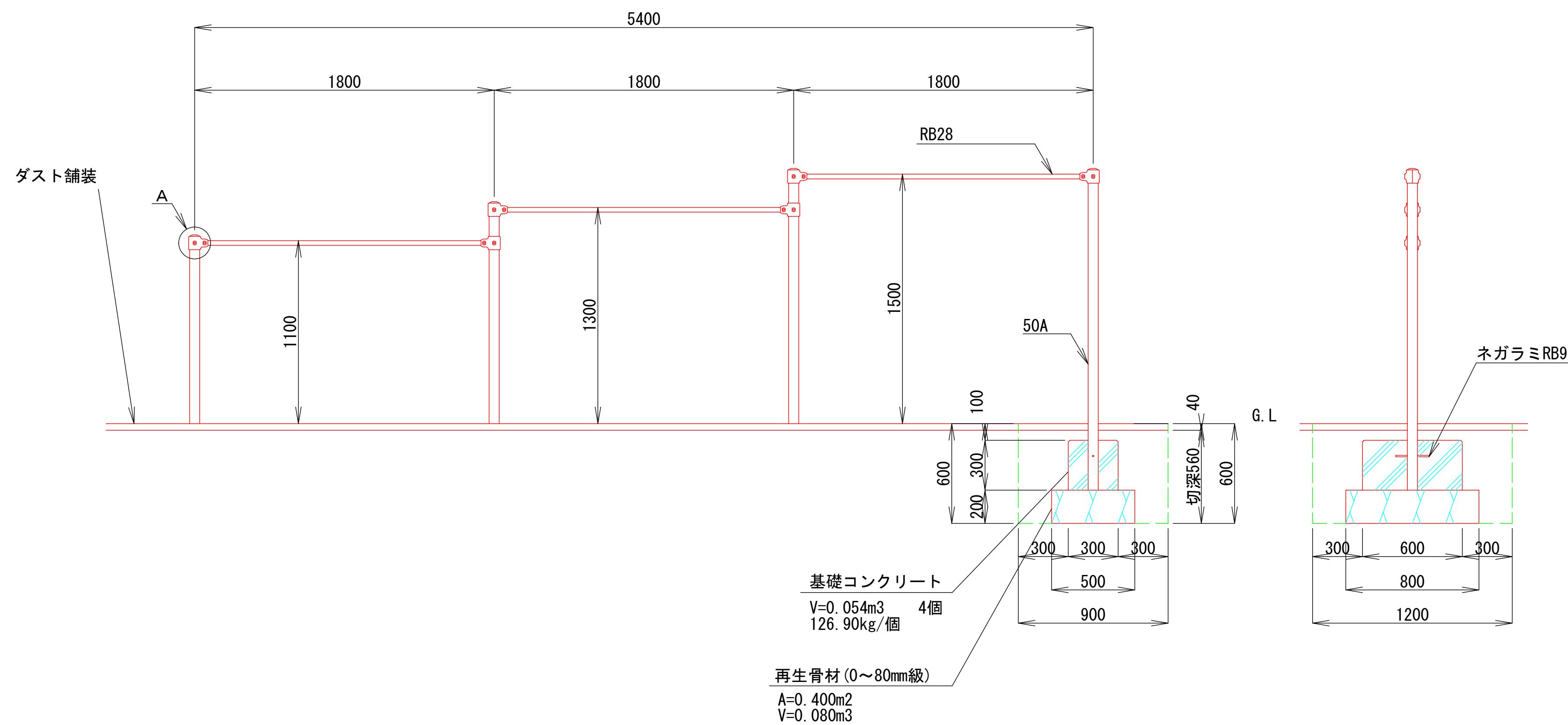
立面図 S=1/20
