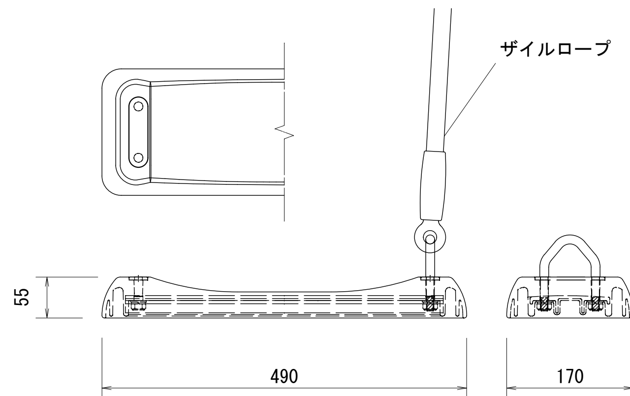
バンパーシート詳細図 S=1:5
