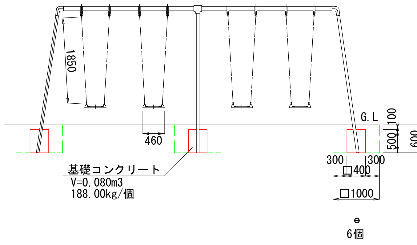
4連ブランコ基礎 1/50
