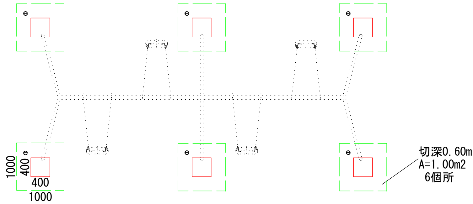
基礎平面図 1/50
