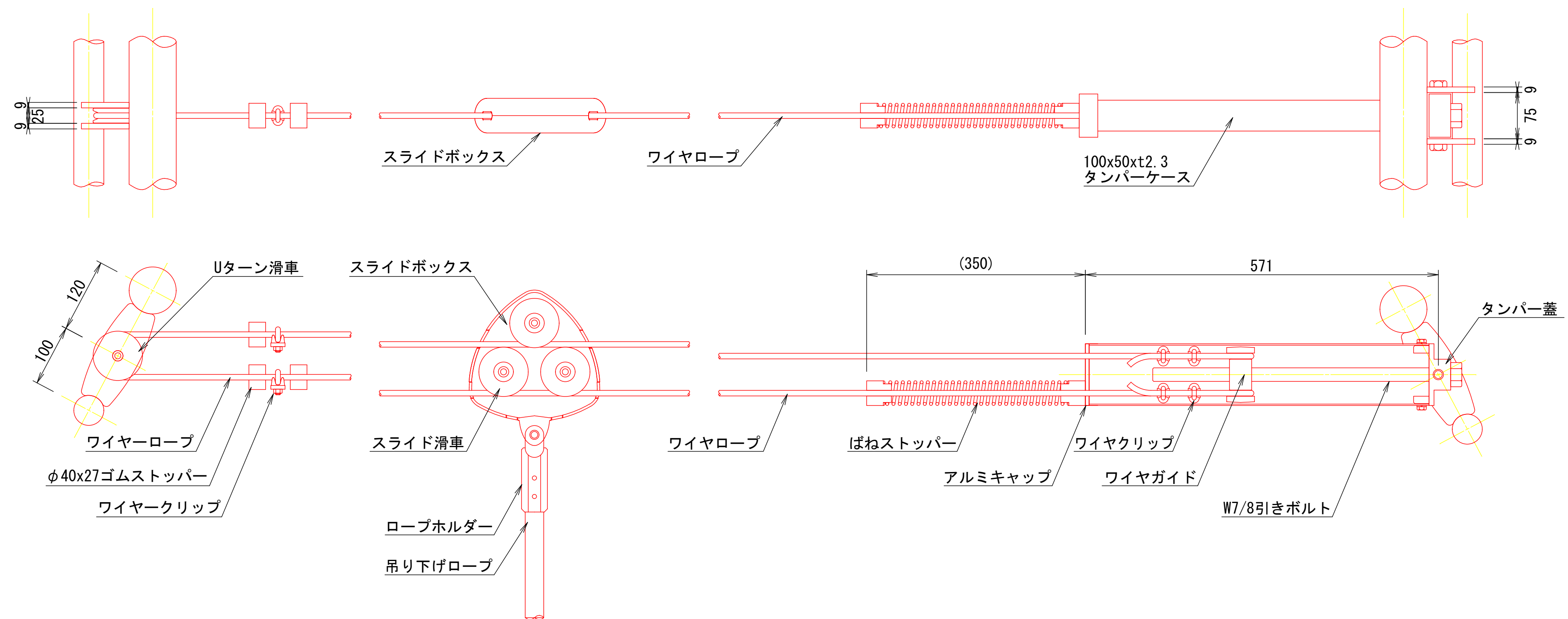
滑走部詳細図 S=1/5
