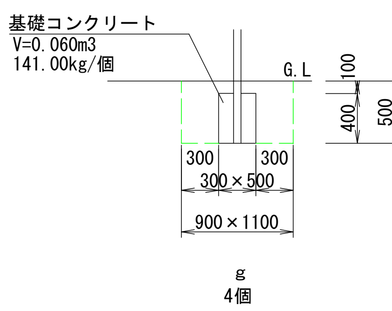
3連低・中鉄棒基礎 1/30
