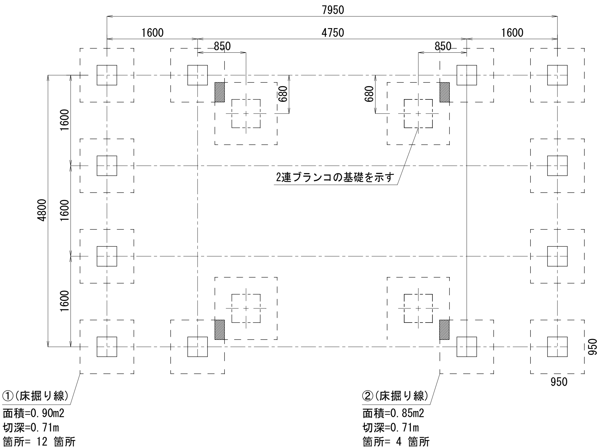
基礎詳細図 S=1:25
