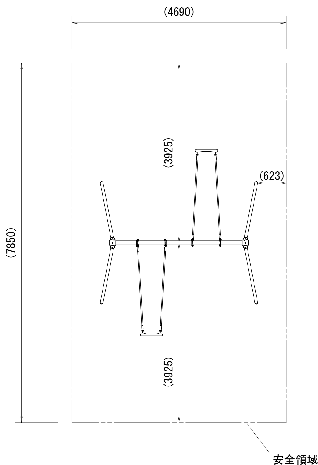
設置スペース S=1:50
