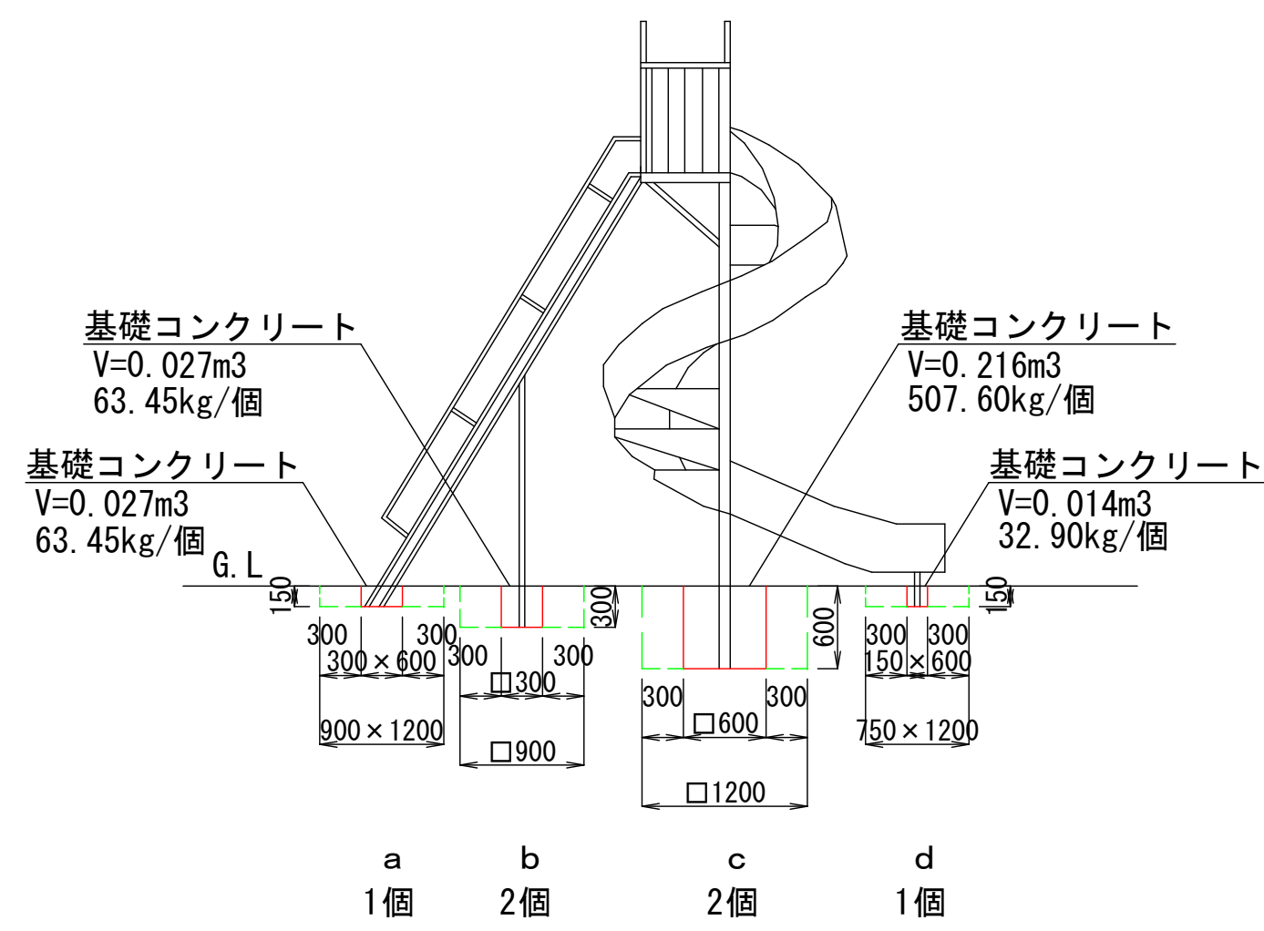
1回転式滑り台基礎 1/50
