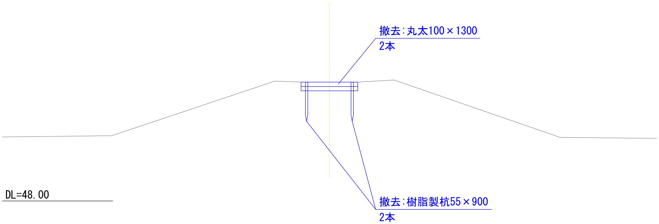
盛土撤去横断面図より
