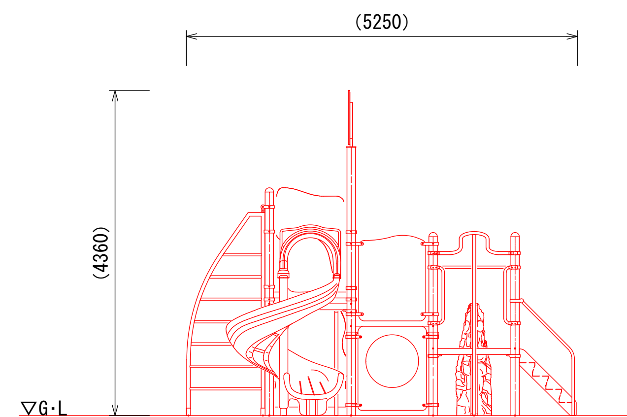
B立面図 S=1/50
