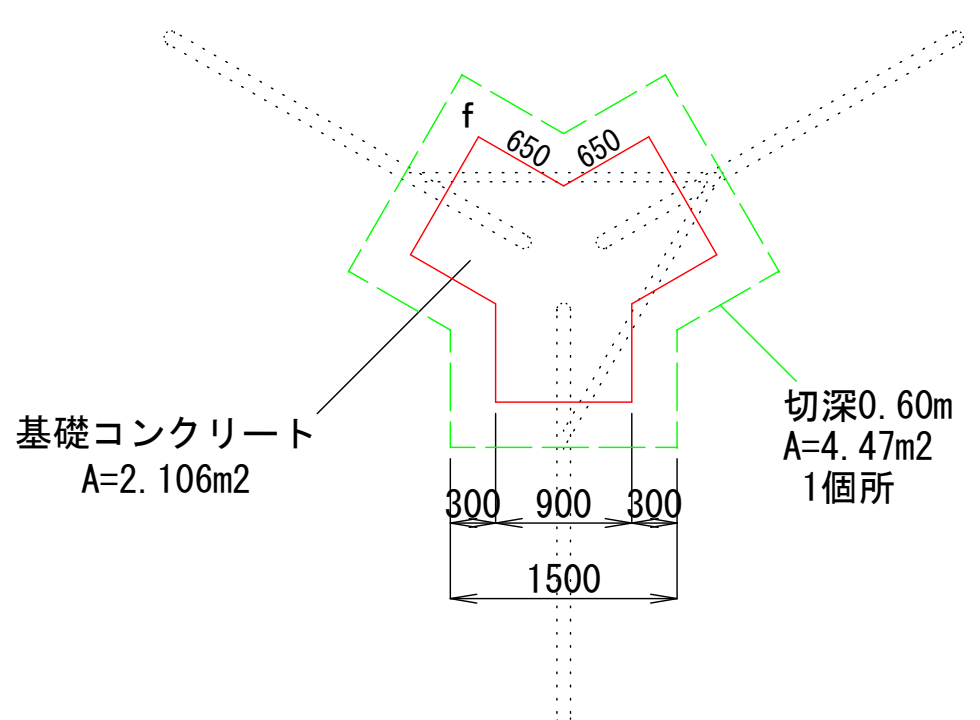
基礎平面図 1/50
