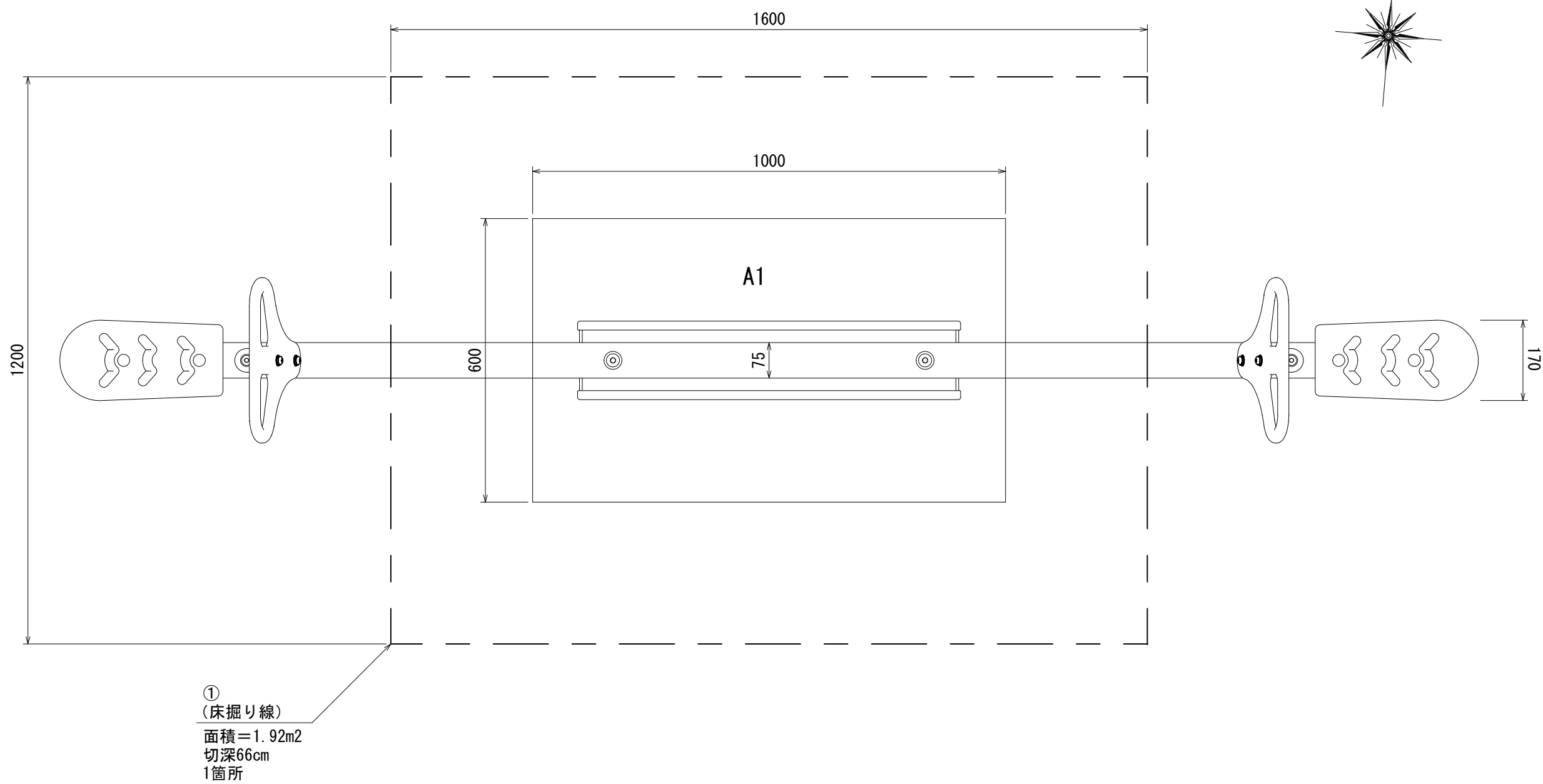
平面図
