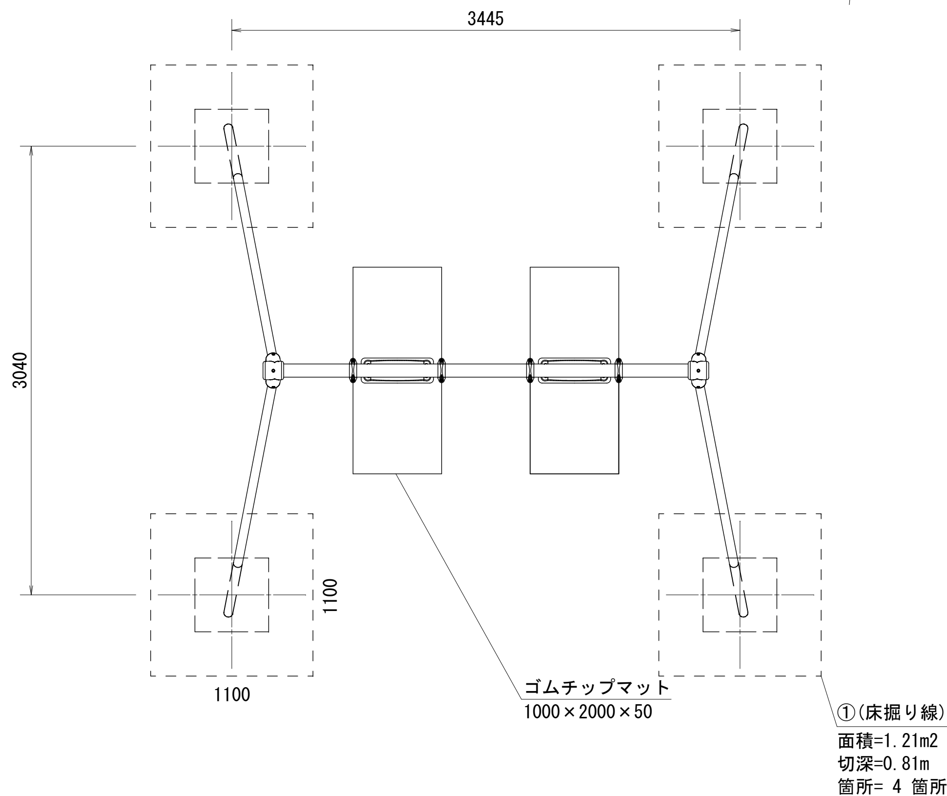
外観図 S=1:25
