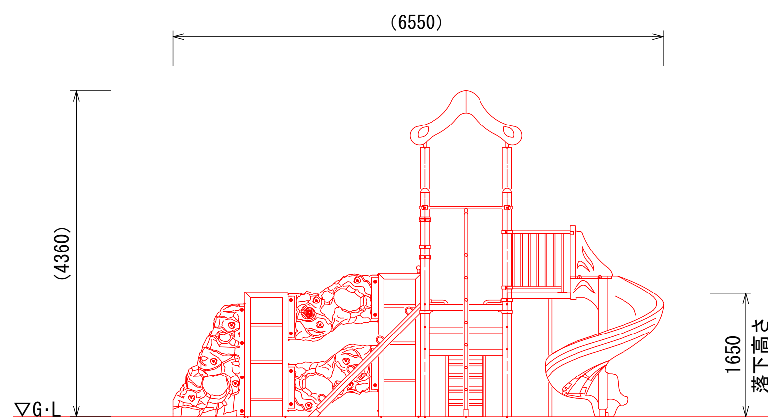
A立面図 S=1/50
