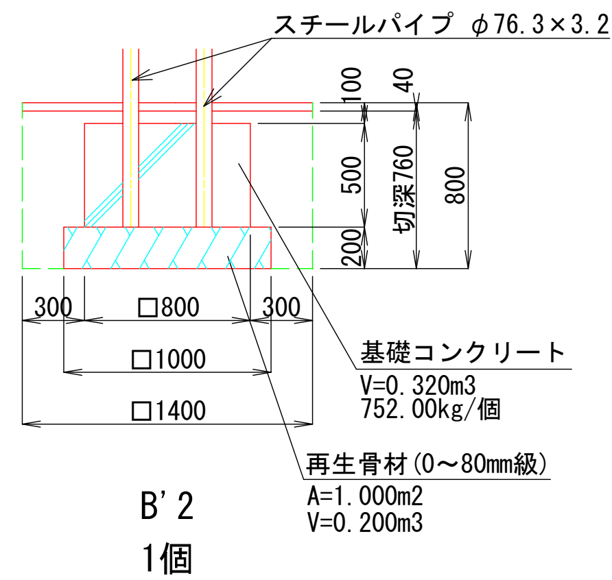
基礎詳細図 S=1/25
