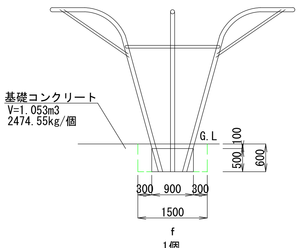
複合遊具基礎 1/50
