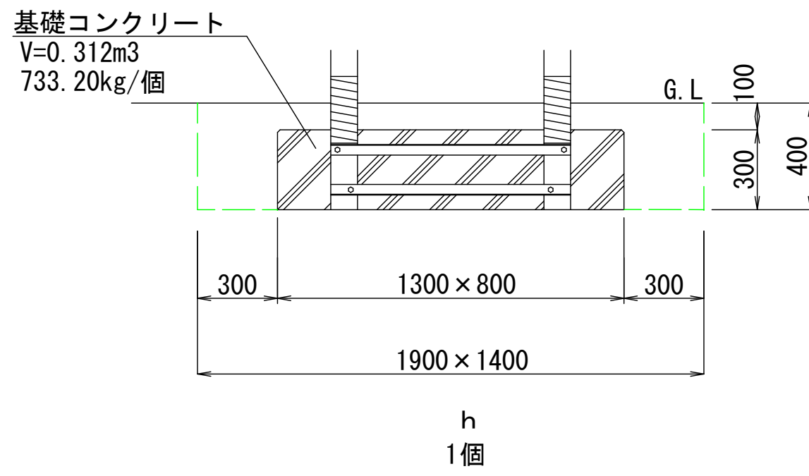
安全ブランコ基礎 1/20
