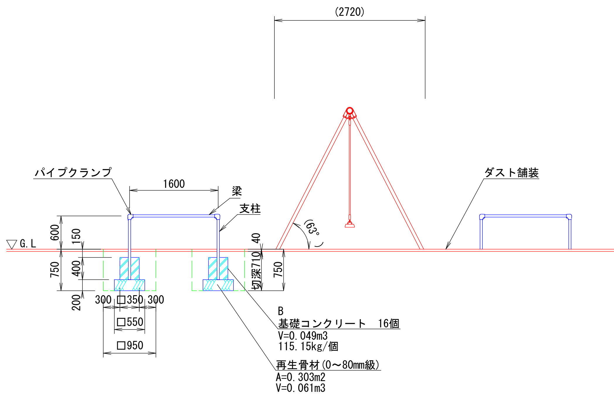
側面図 S=1/40
