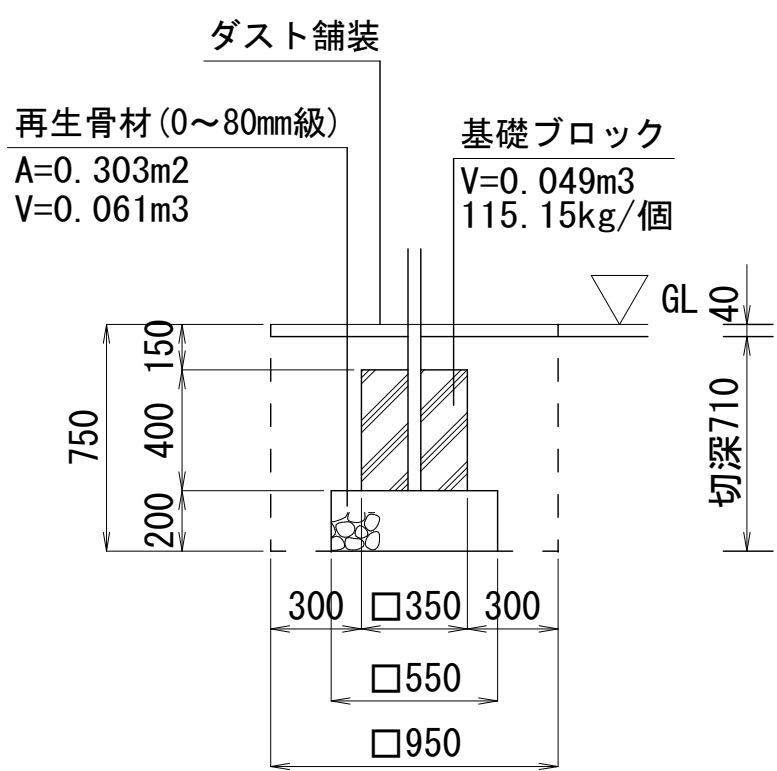
基礎B (12個)
