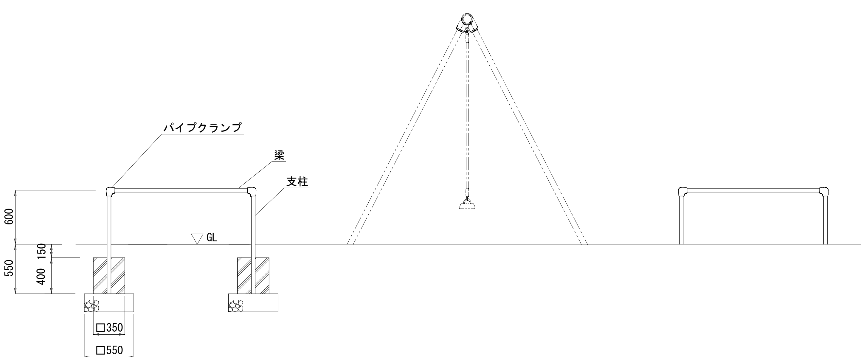
立面図 S=1:25
