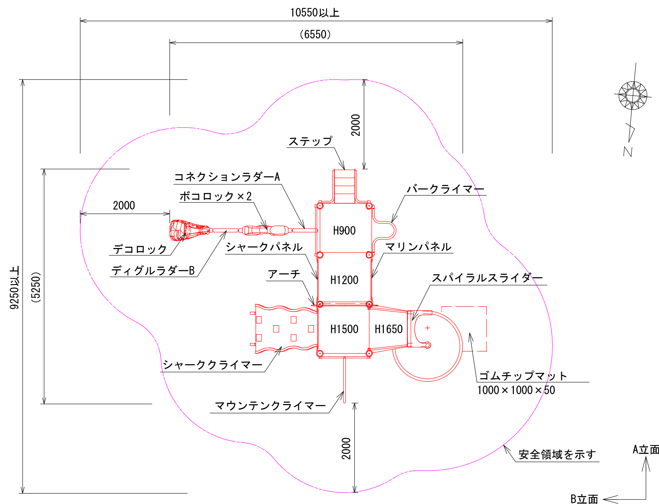
平面図 S=1/50
