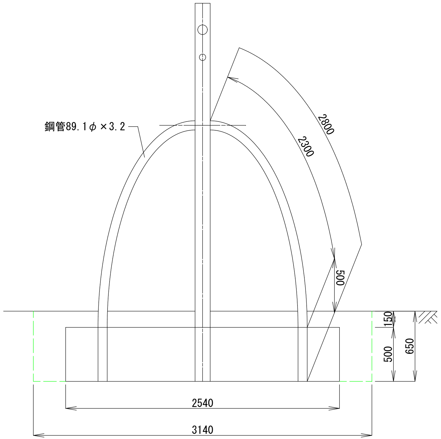
側面図
