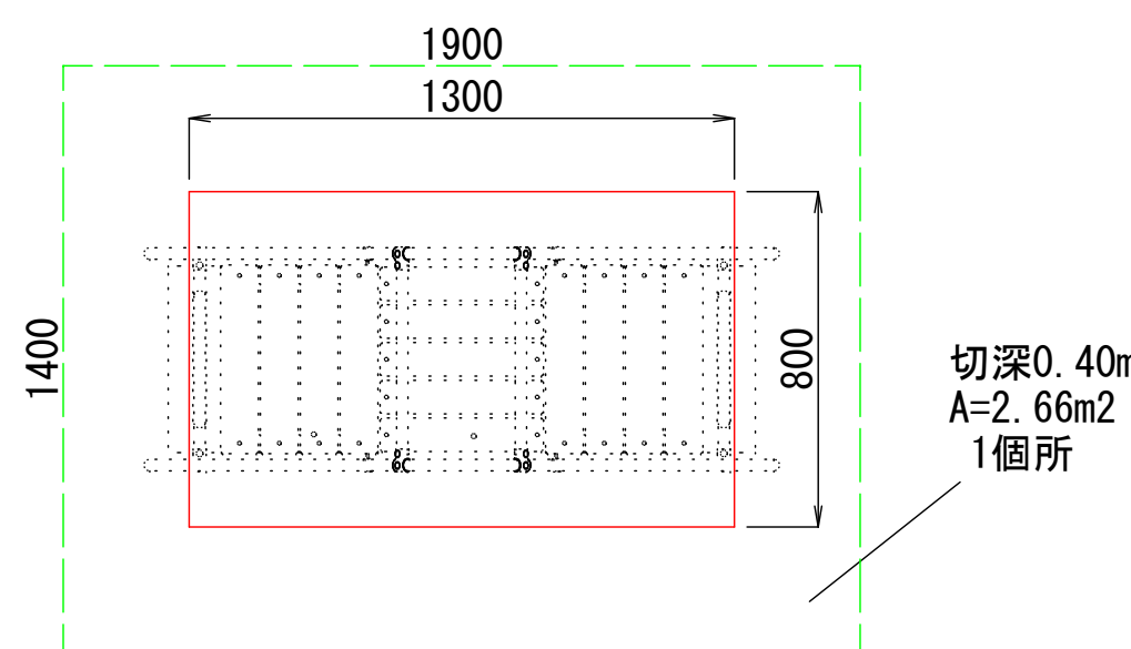
基礎平面図 1/20
