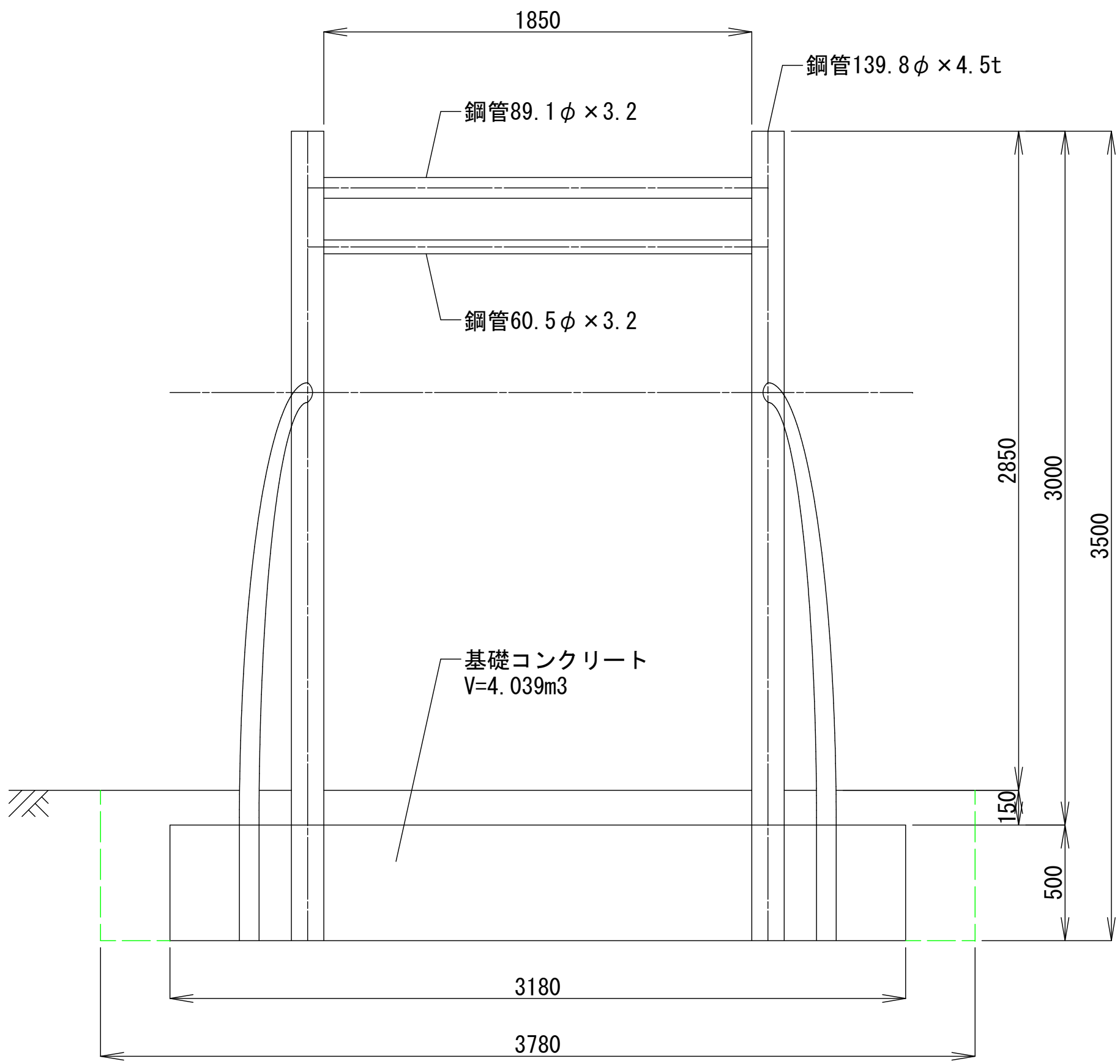
正面図
