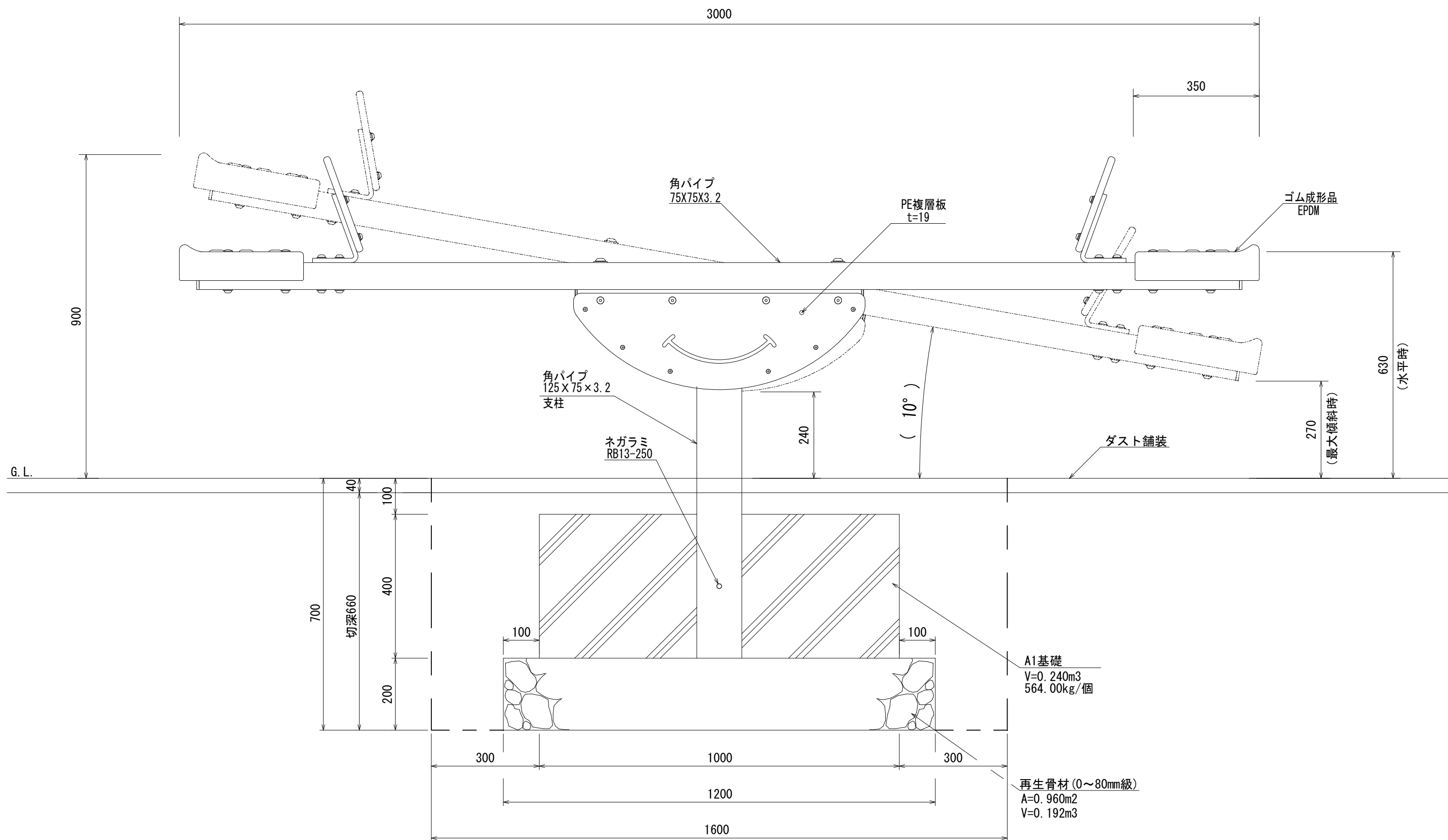
側面図
