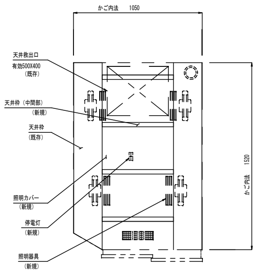
天井伏図
