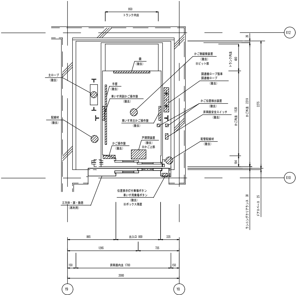
昇降路平面図
