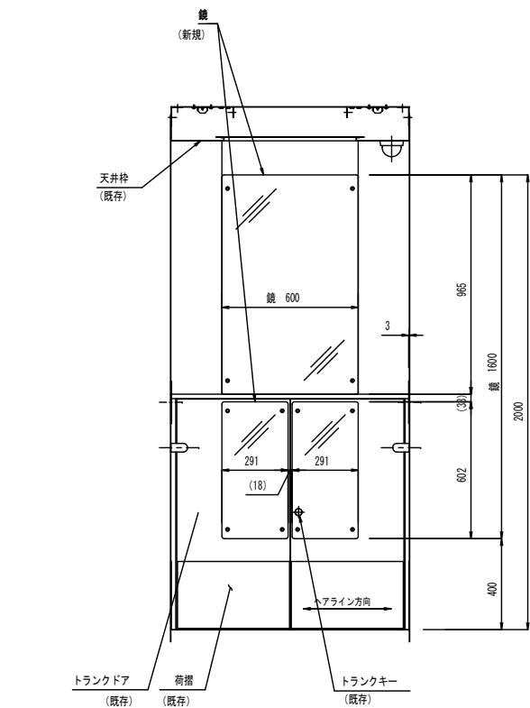
背面図
