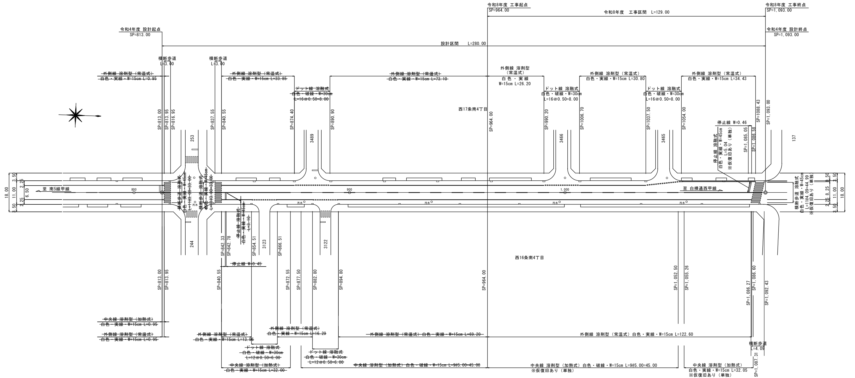
区画線工図 S=1:500
