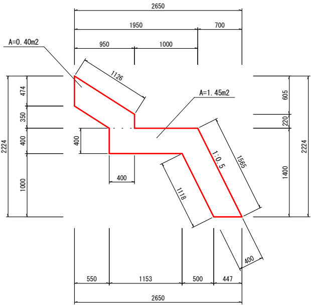
A-A 断面詳細図 S=1:30
