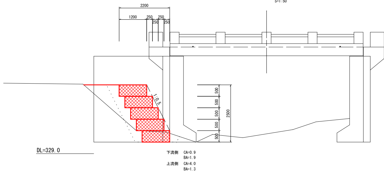
側面図 S=1:50
