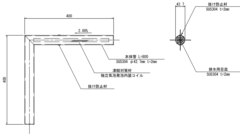
水抜きパイプ詳細図 S=1:5
