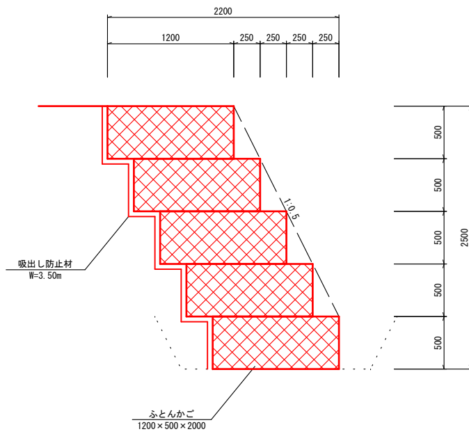
ふとんかご詳細図 S=1:25
