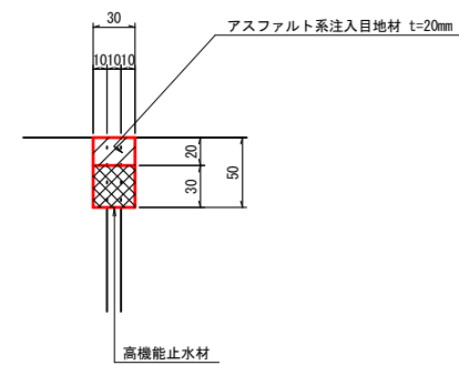
A2橋台部 断面詳細図
