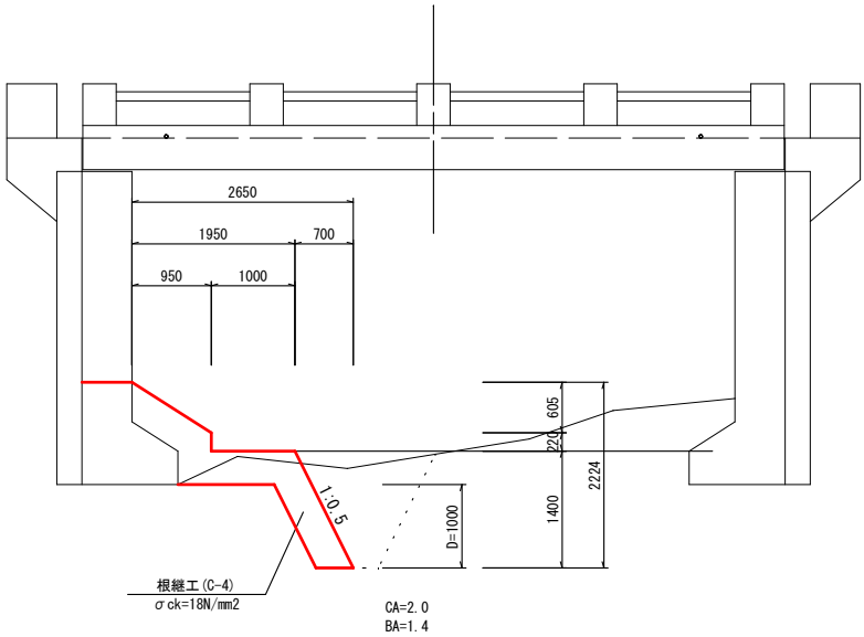
側面図 S=1:50
