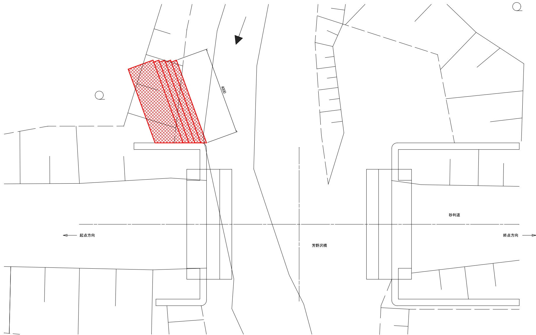
平面図 S=1:50
