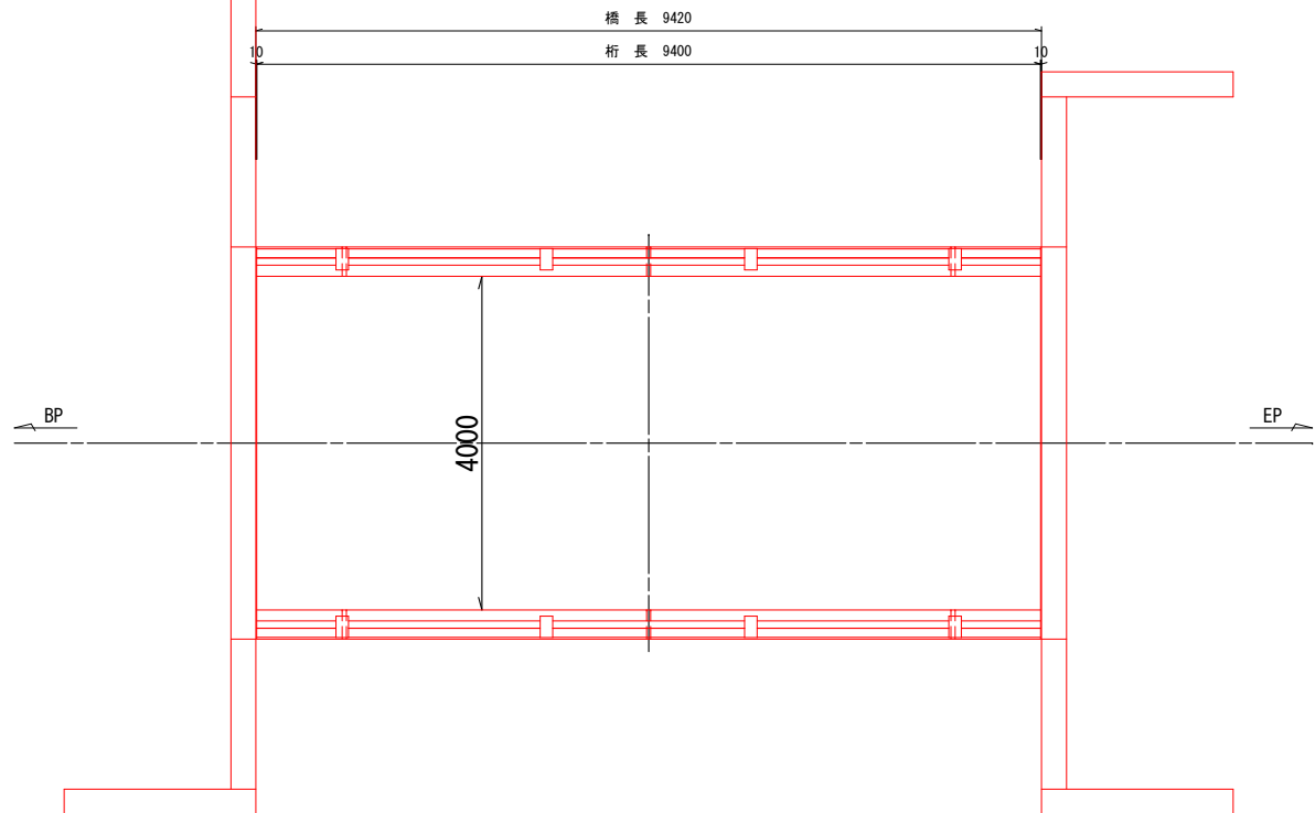
平 面 図 S=1:50
