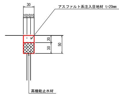
A1橋台部 断面詳細図
