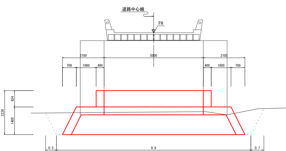
正面図 S=1:50
