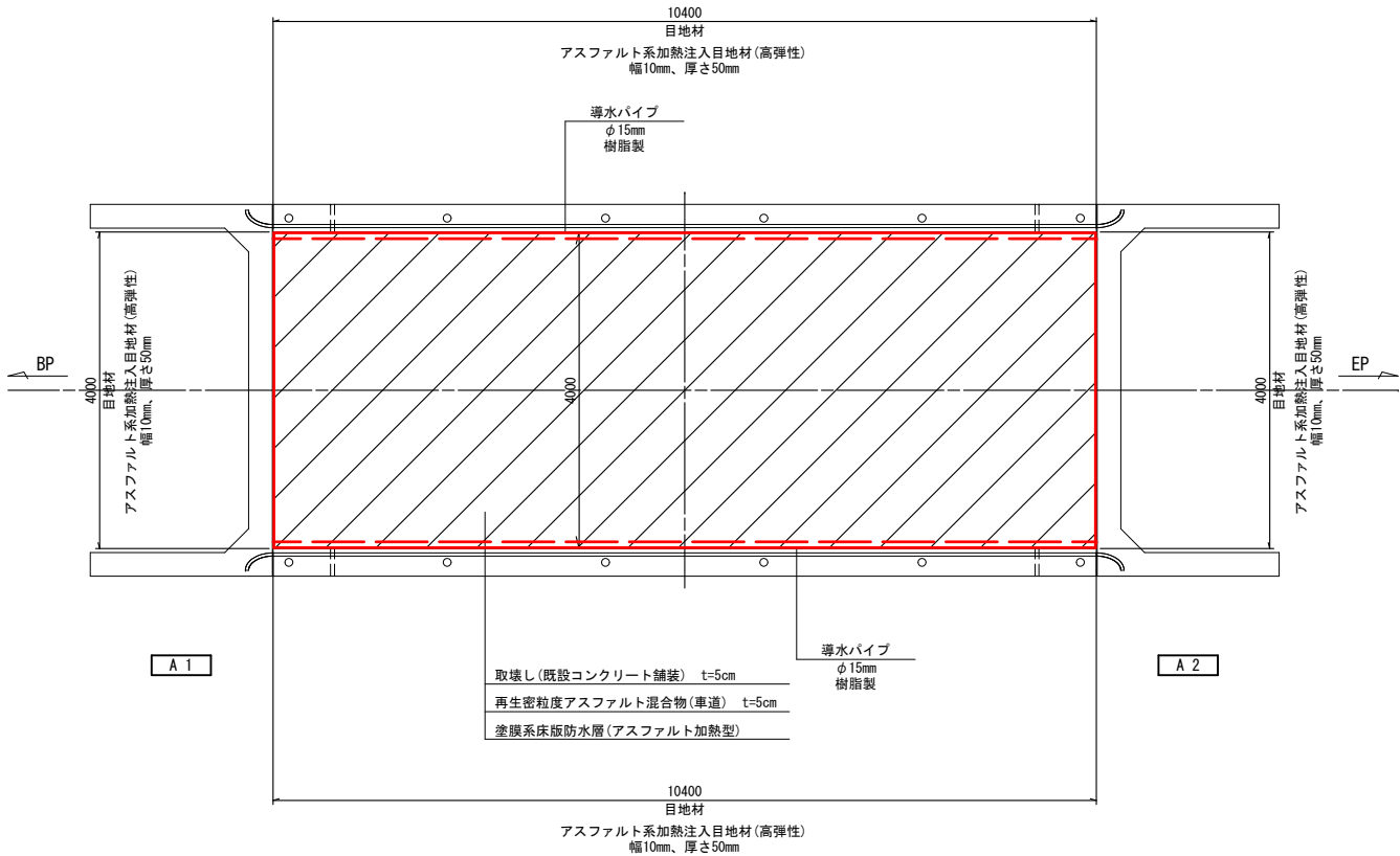
平面図 S=1:50
