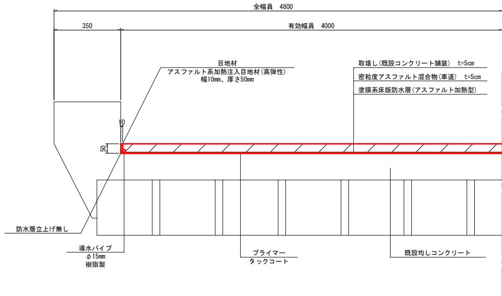
伸縮装置部 S=1:10
