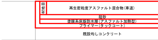
層構成概要図
