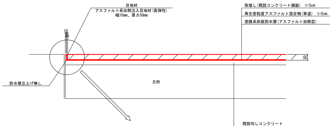
層構成概要図
