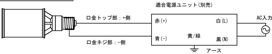
LEDランプ結線図
