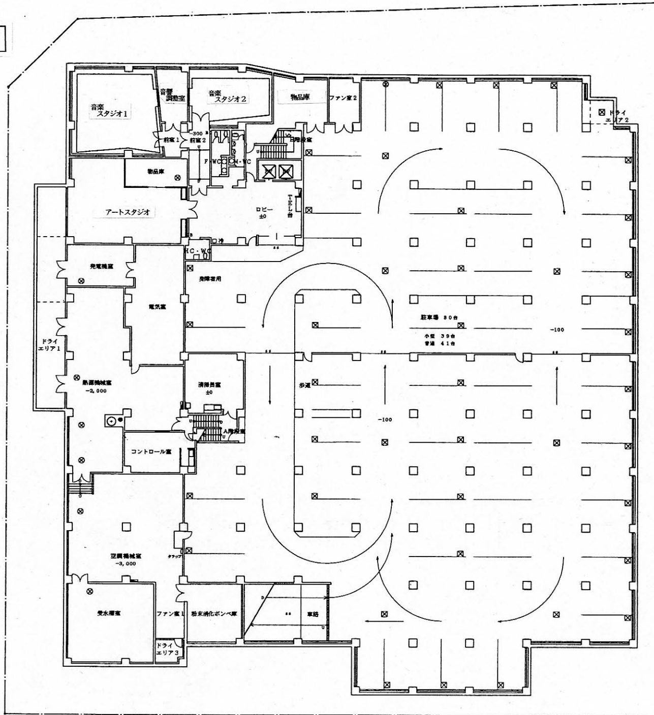
とまちプラザ地階平面図
