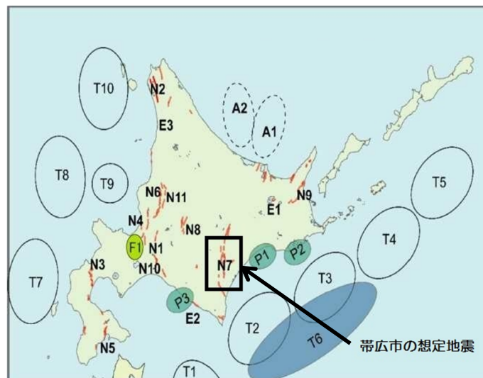
北海道における想定地震 [北海道地域防災計画抜粋]
