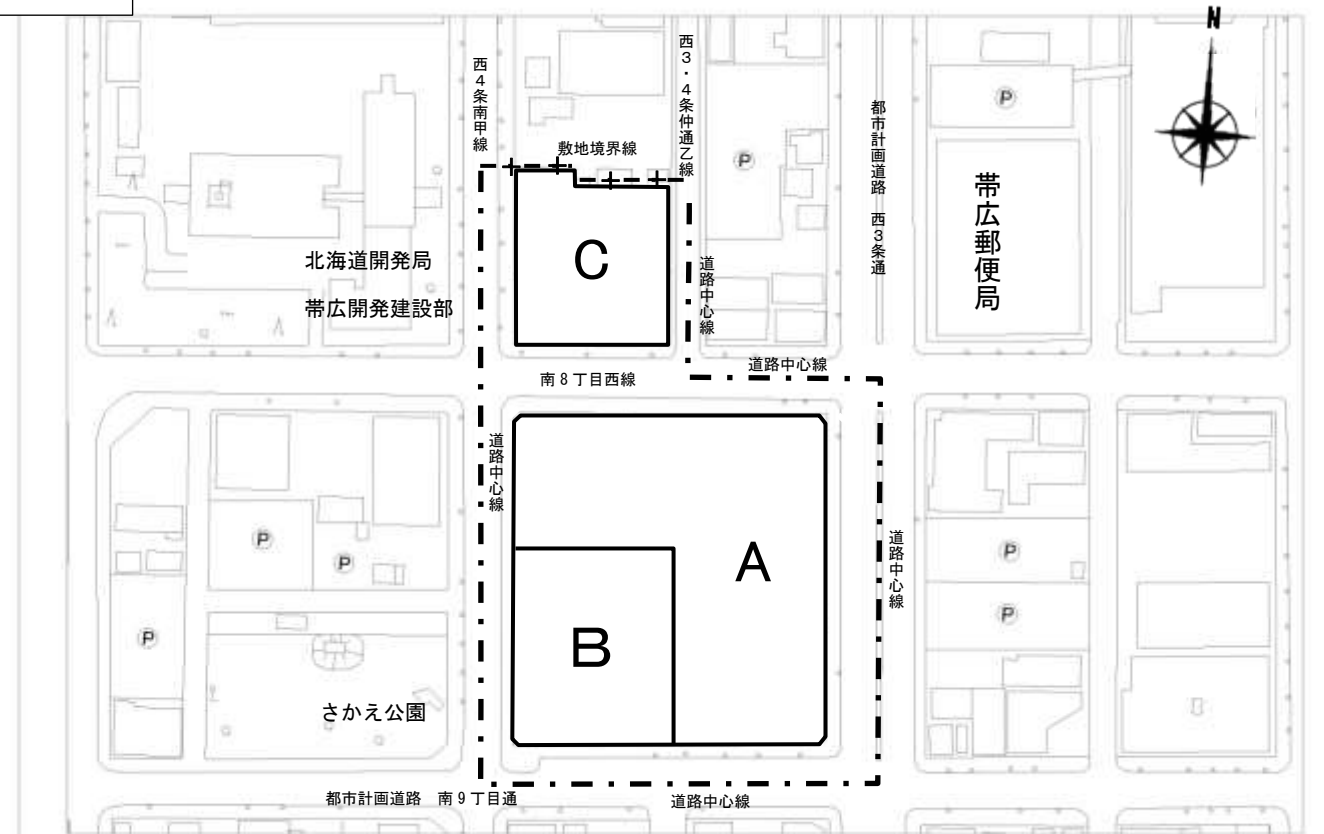
計画図
