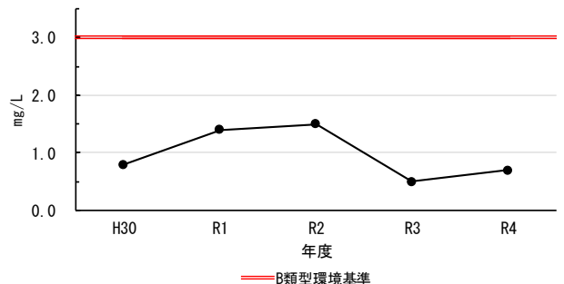
札内川 (浄水場取水口) のBOD (75%値) 経年変化
