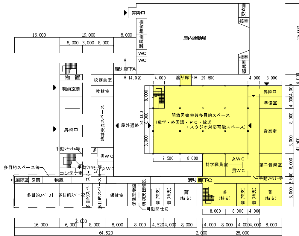
1F 増築・改修後平面図 (案)
