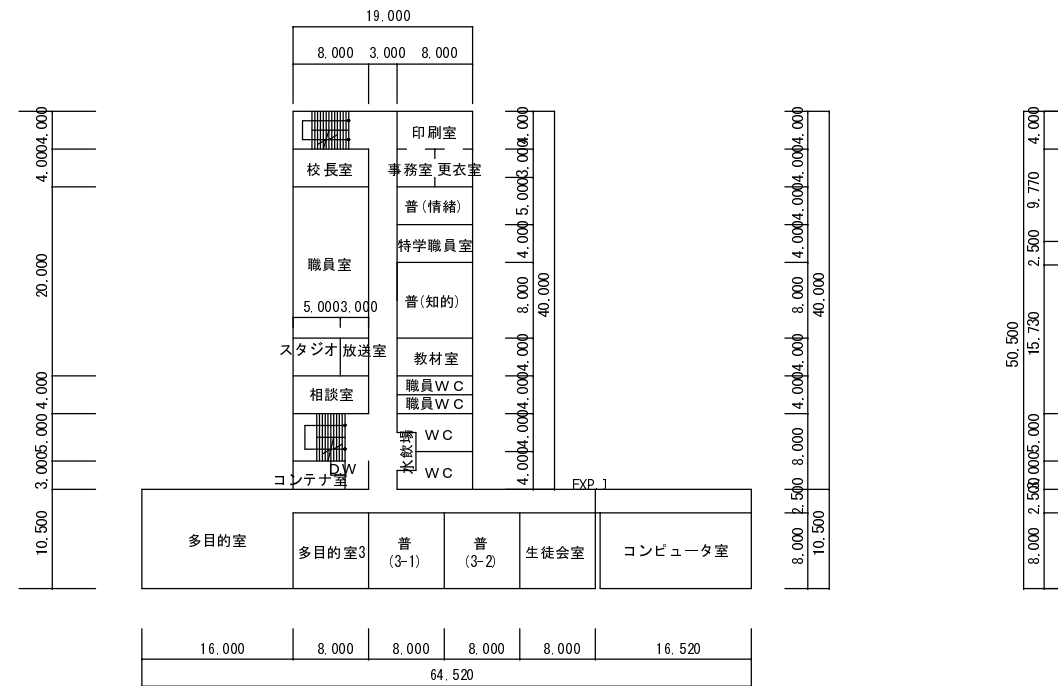
2F 現況平面図
