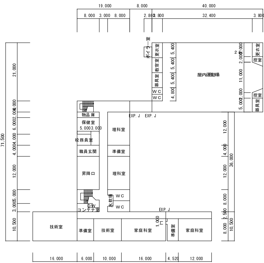
1F 現況平面図
