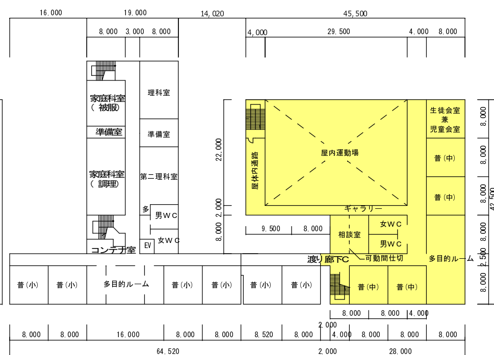
3F 増築・改修後平面図 (案)
