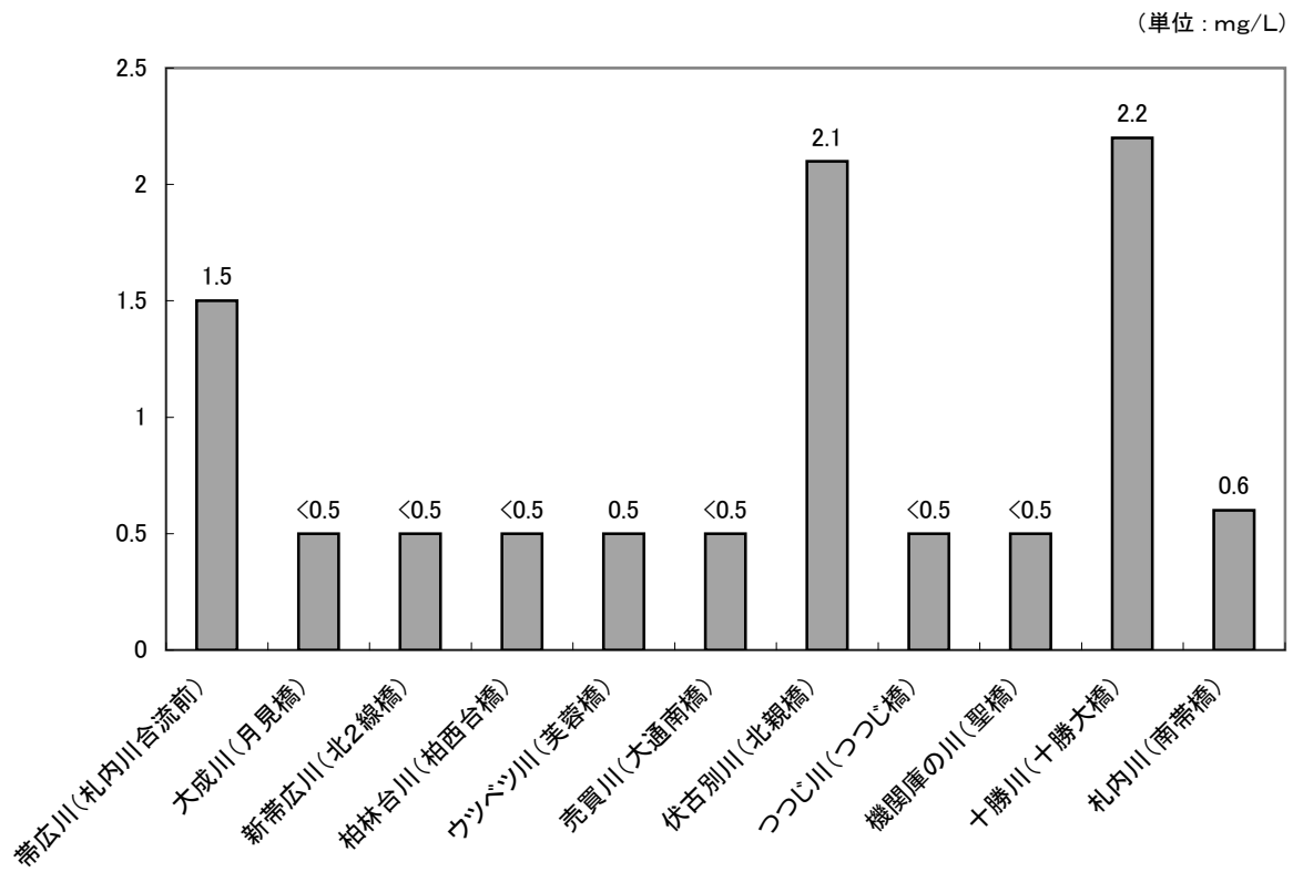
河川汚濁度(BOD測定結果) (平成22年度)
