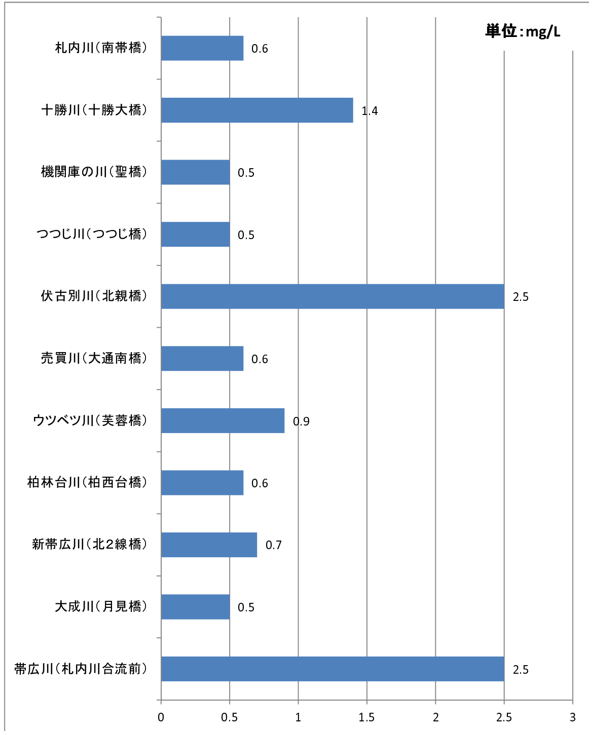
河川汚濁度(BOD測定結果) (平成27年度)
