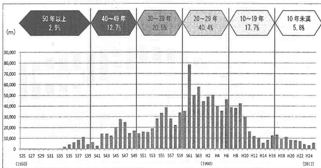
図10 下水道管の年度別整備延長
