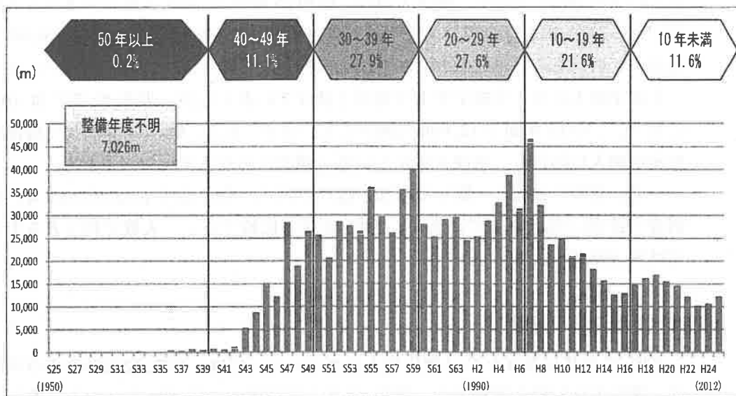
図9 水道管の年度別整備延長
