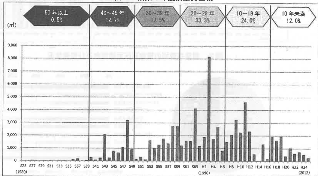
図5 橋梁の年度別整備面積
